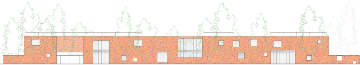
délnyugati homlokzat m 1:200
