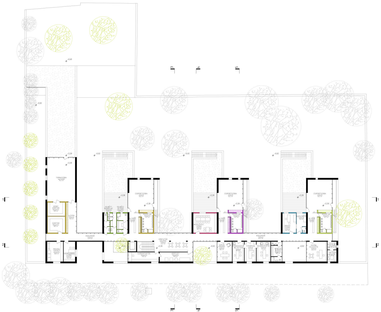
emeleti alaprajz m 1:200
