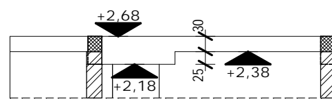
KOSZORÚ METSZET
