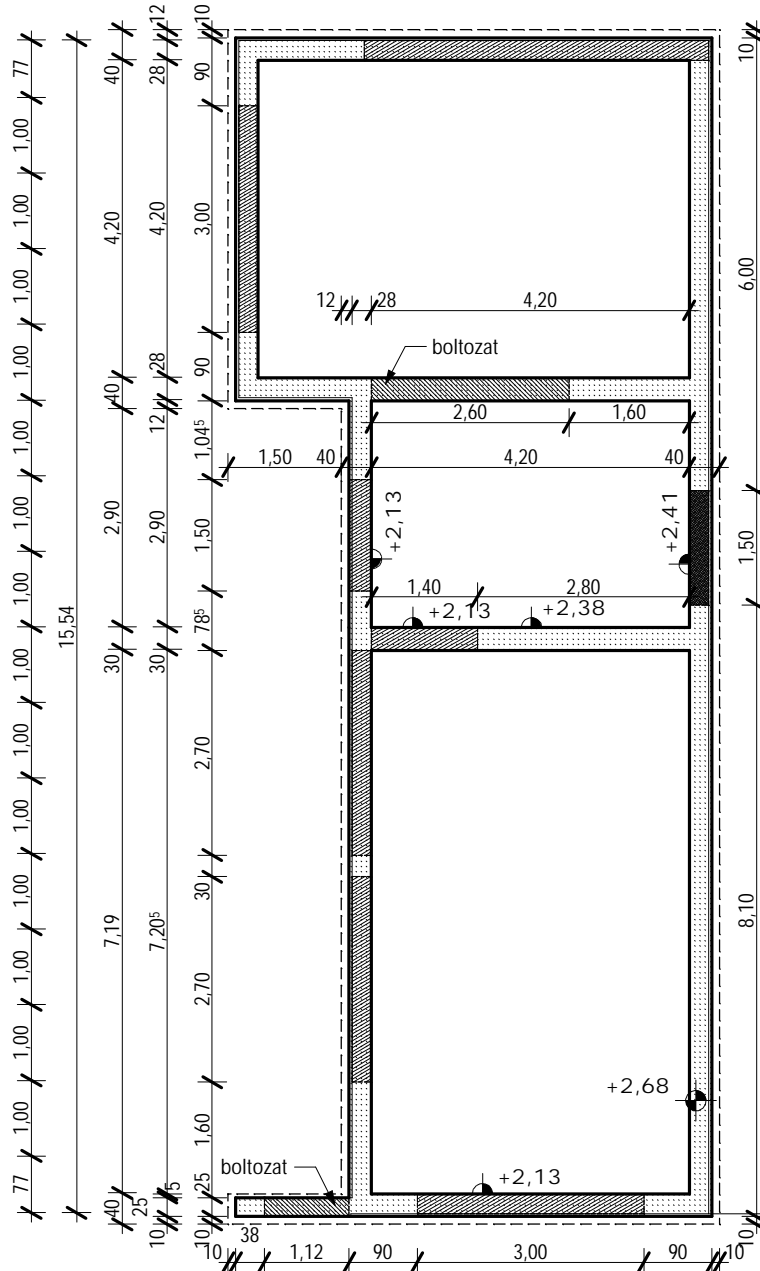
KOSZORÚ ALAPRAJZ
