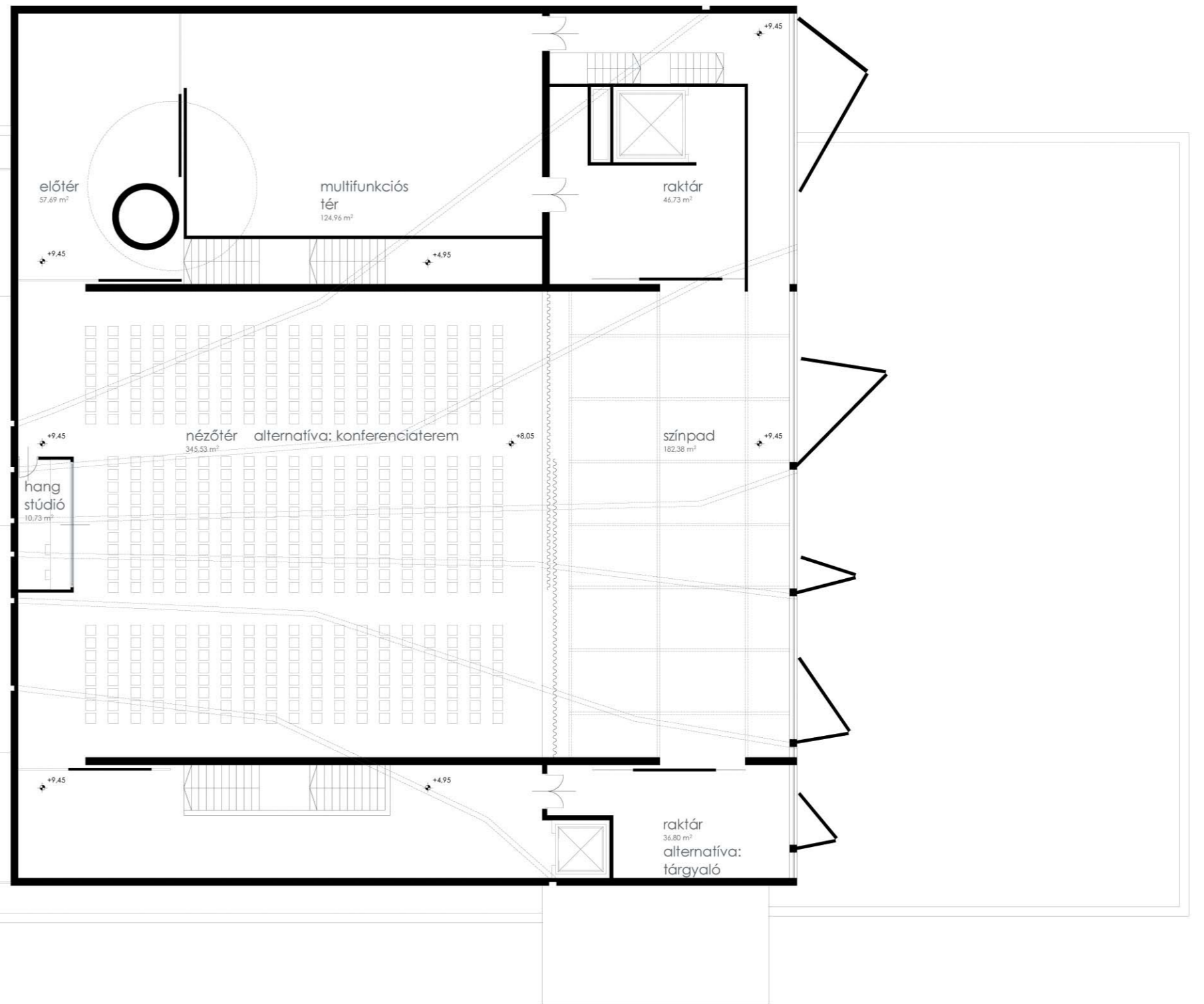
2. emeleti alaprajz m=1:200
