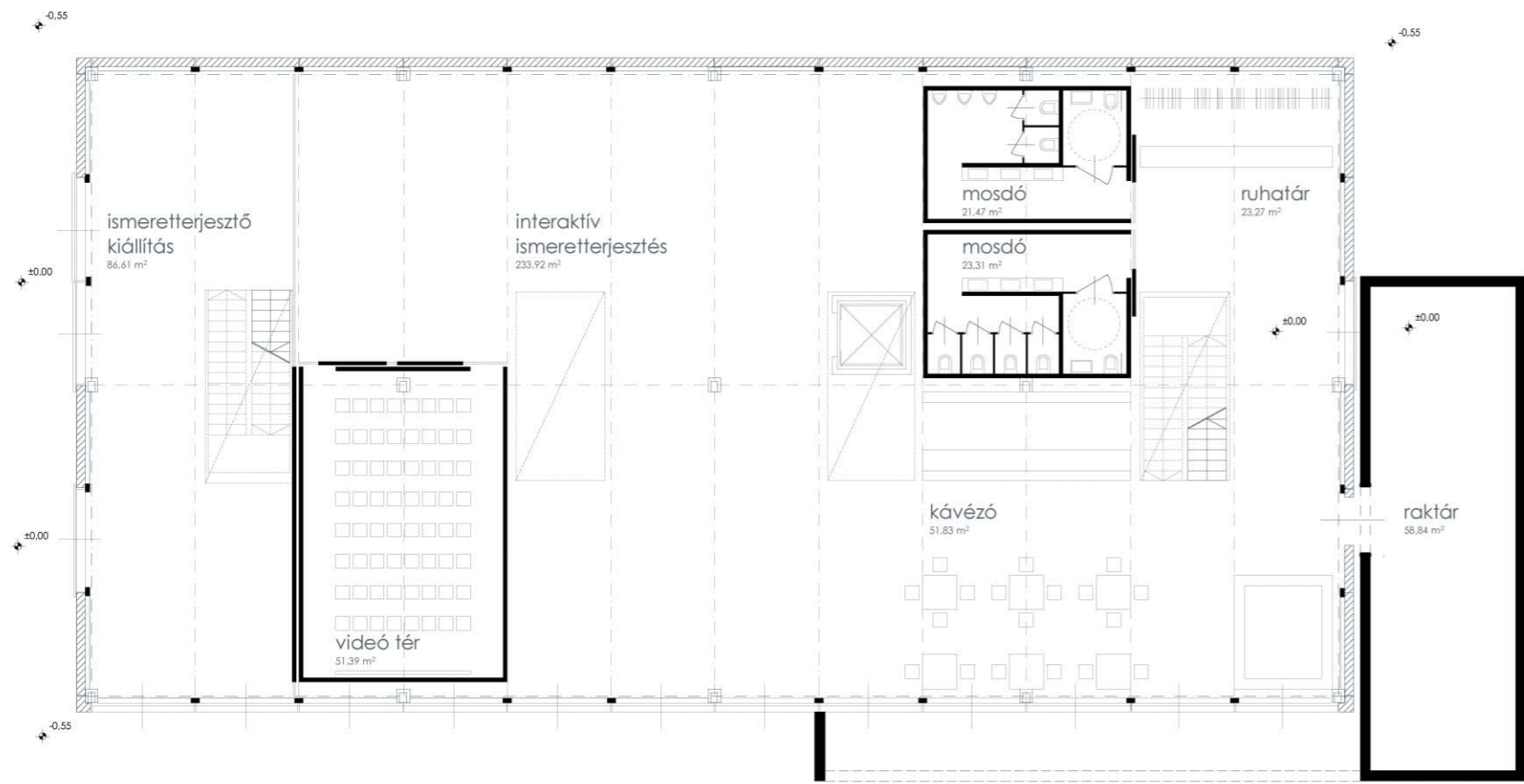
tudásház földszinti alaprajz m=1:200
