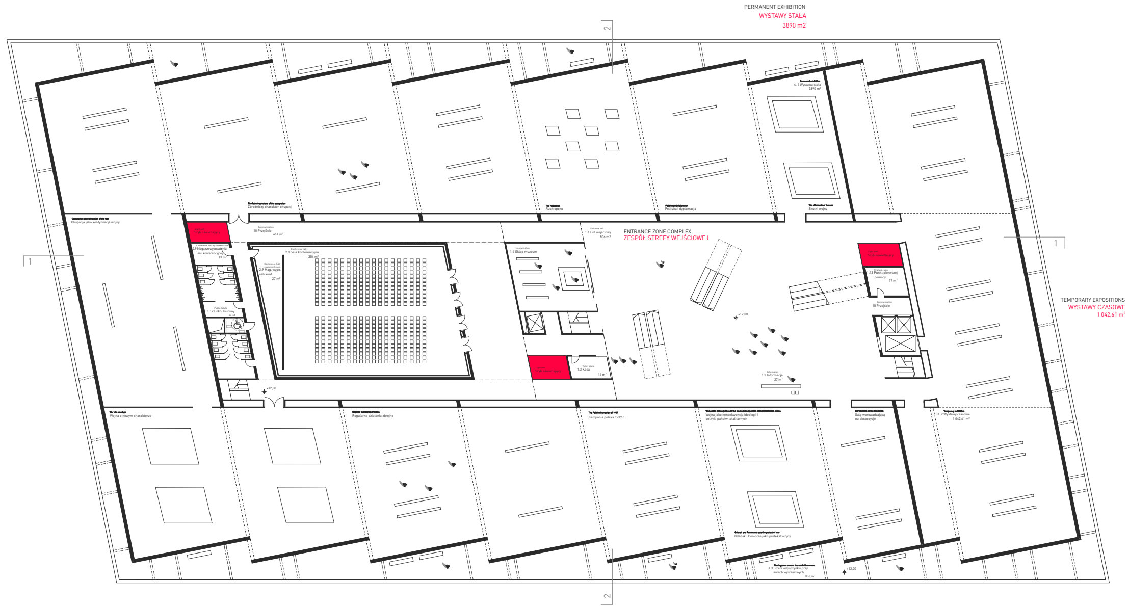
0 10 1ST FLOOR PLAN RZUT 1. PIĘTRA 1:200
