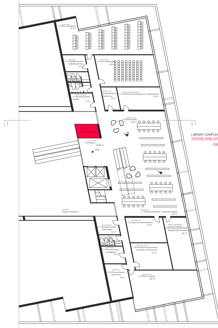
2 ST FLOOR PLAN / B RZUT 2. PIĘTRA / B 1:200
