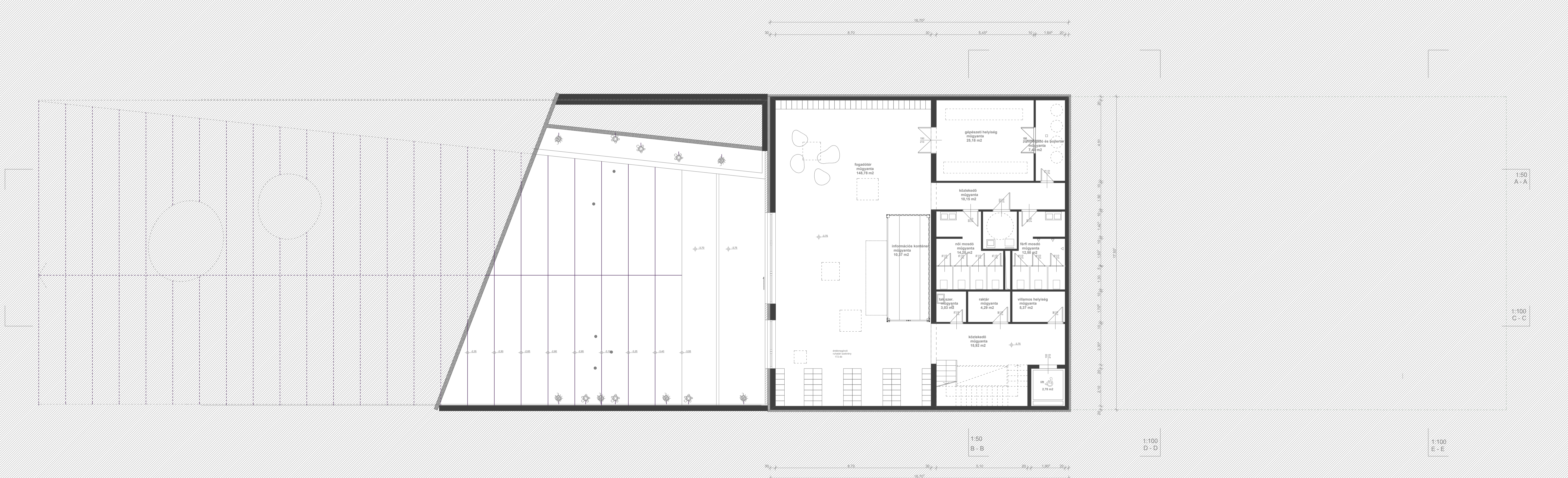
5 PINCESZINTI ALAPRAJZ m = 1 : 100
