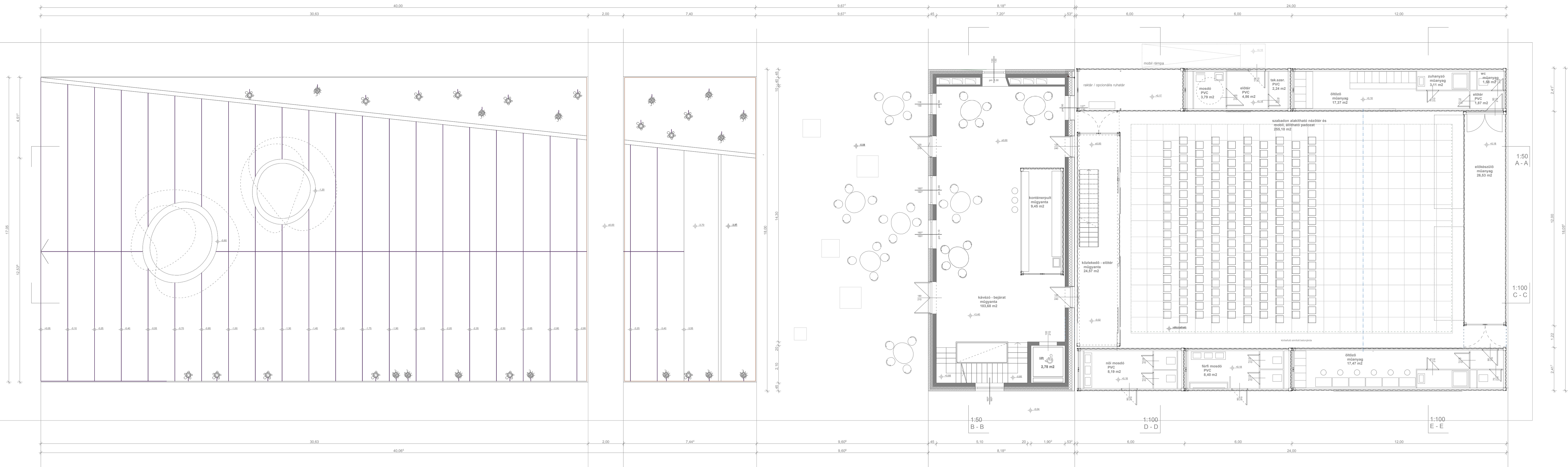
6 FÖLDSZINTI ALAPRAJZ m = 1 : 100
