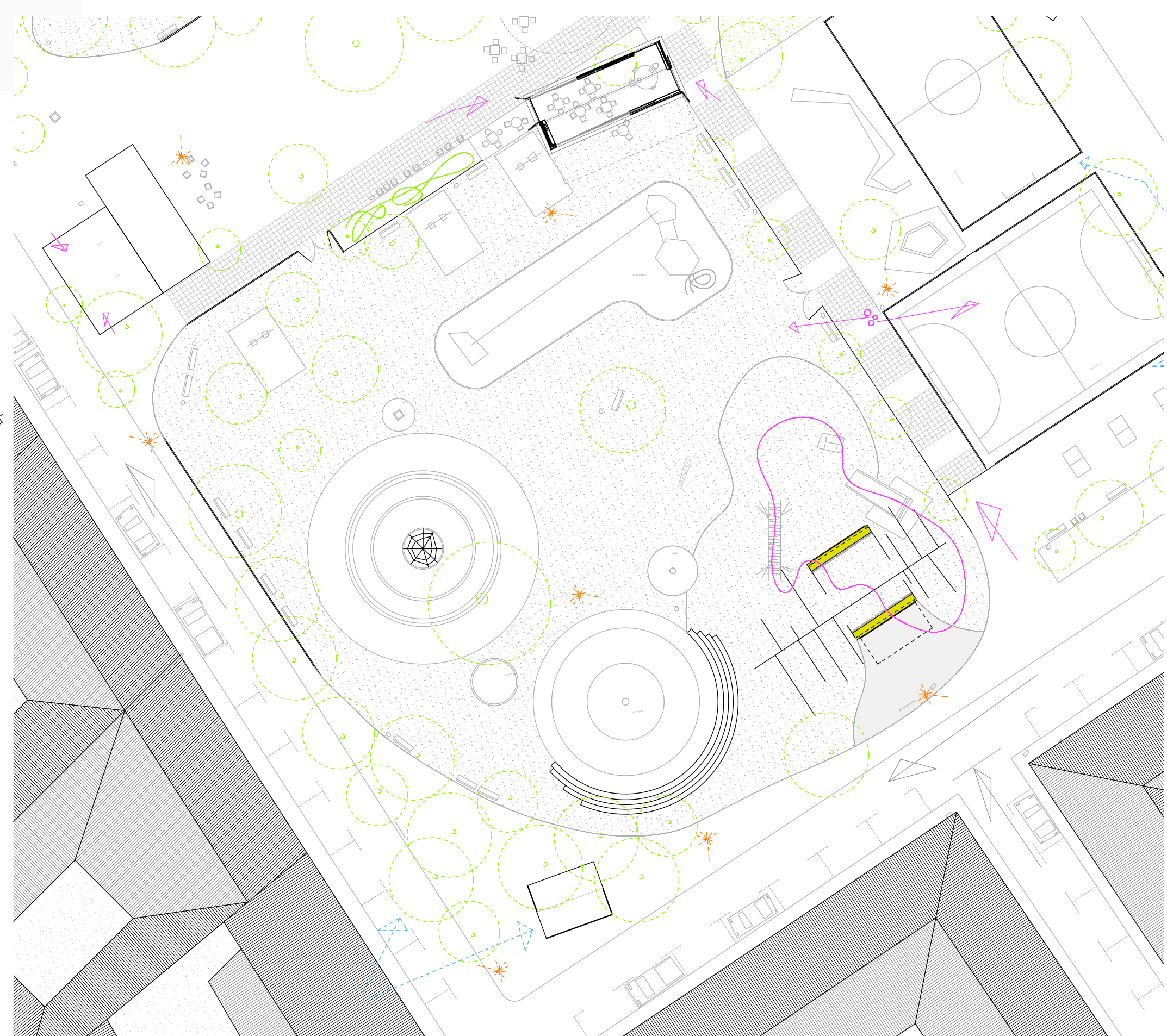
helyszínrajz m=1:350
