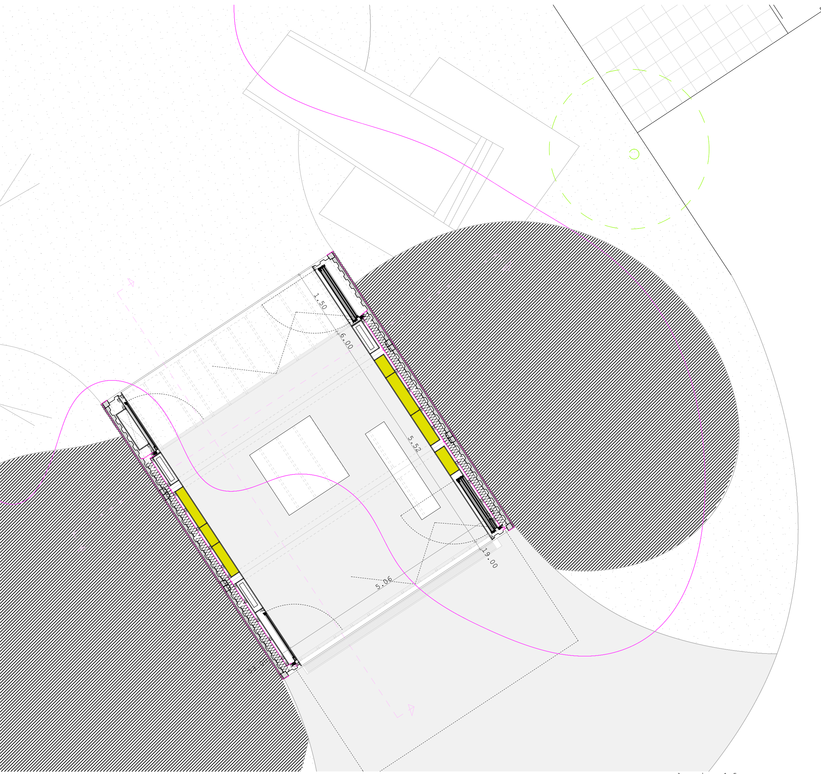
alaprjz m=1:50
