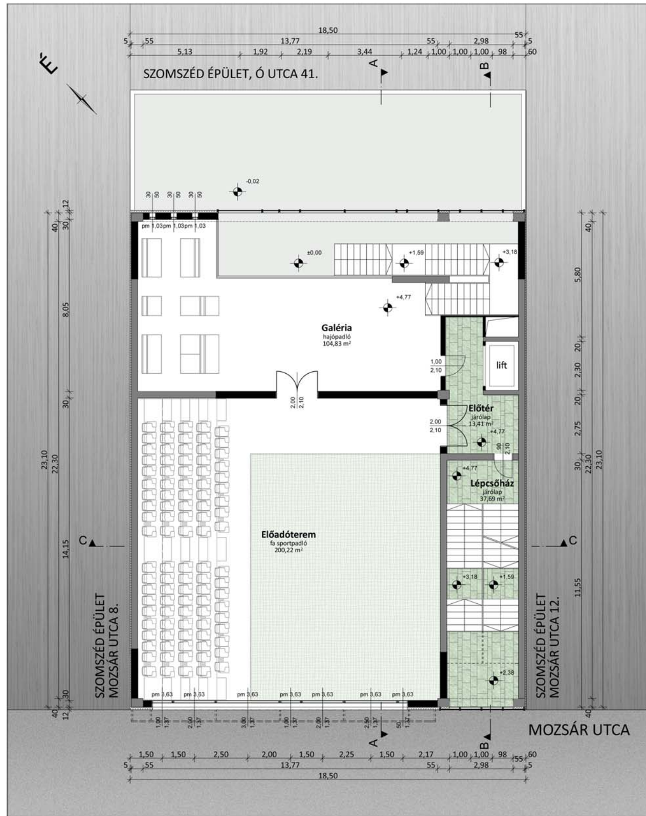
1. EMELET ALAPRAJZA M=1:100
