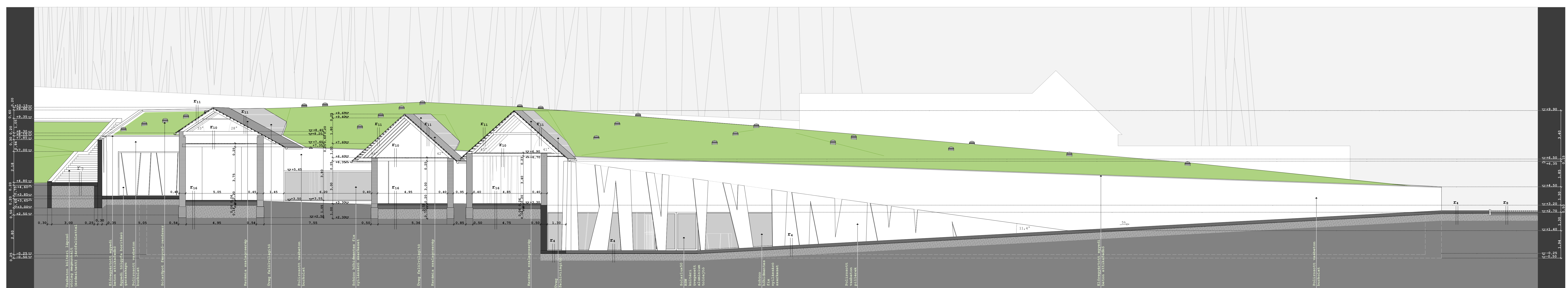
G-G metszet m=1:100
