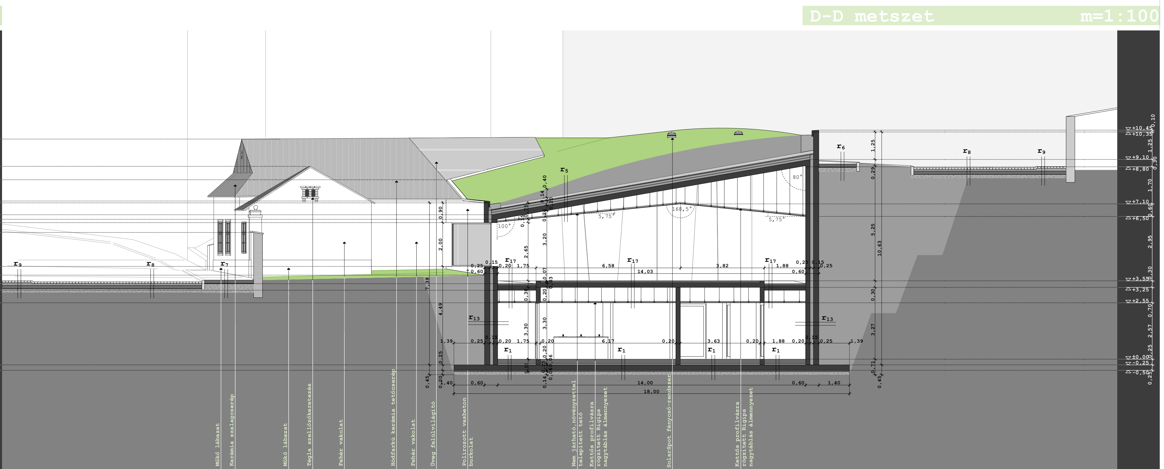
C-C metszet m=1:100
