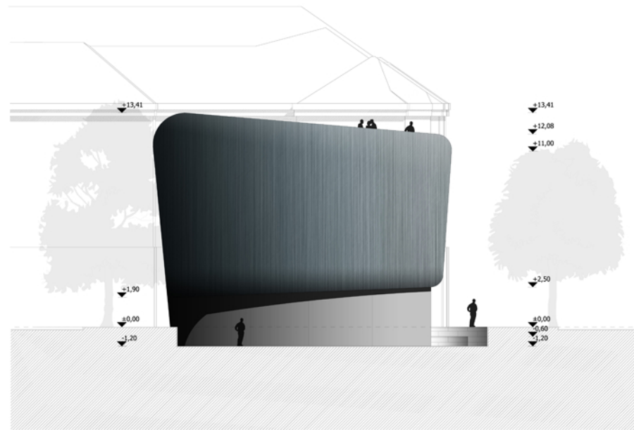
Északi homlokzat M 1:100
