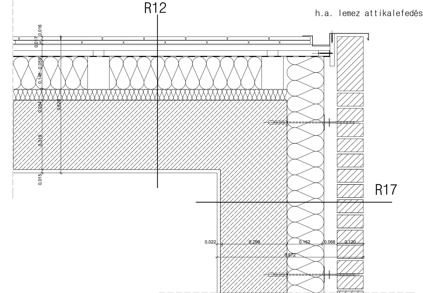
oromfal csatlakozás
