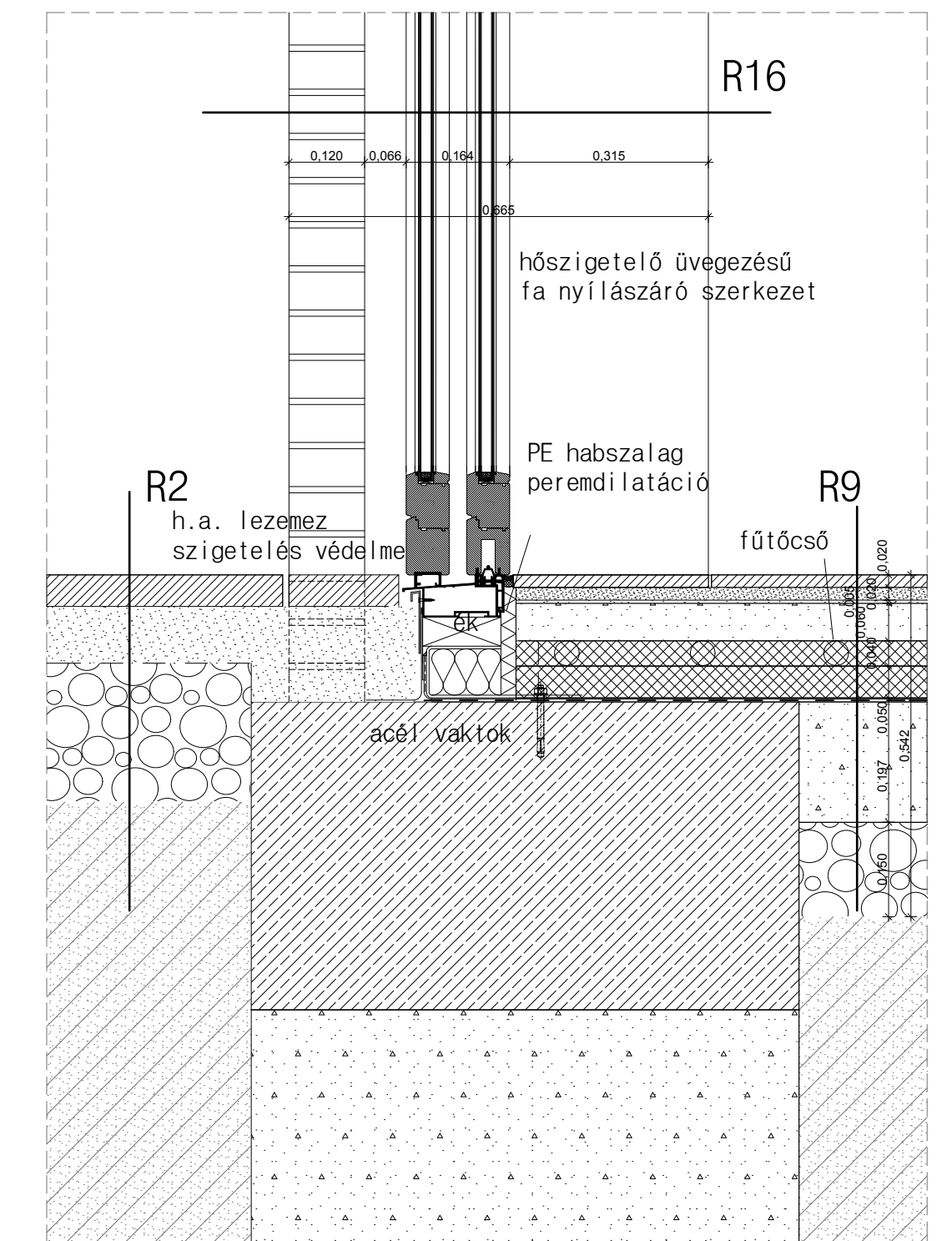
lábazat pince nélkül
