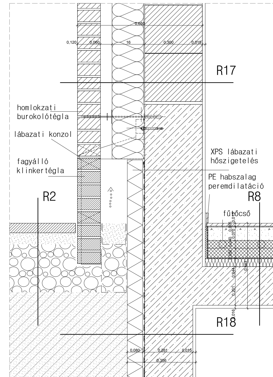
lábazati csomópont pincével
