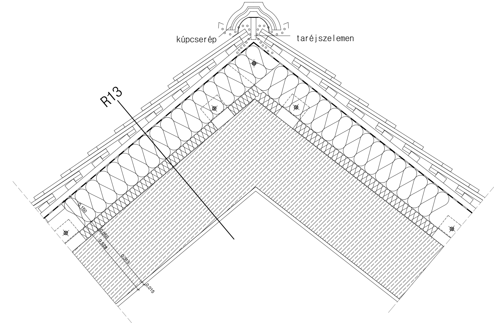
gerinc
