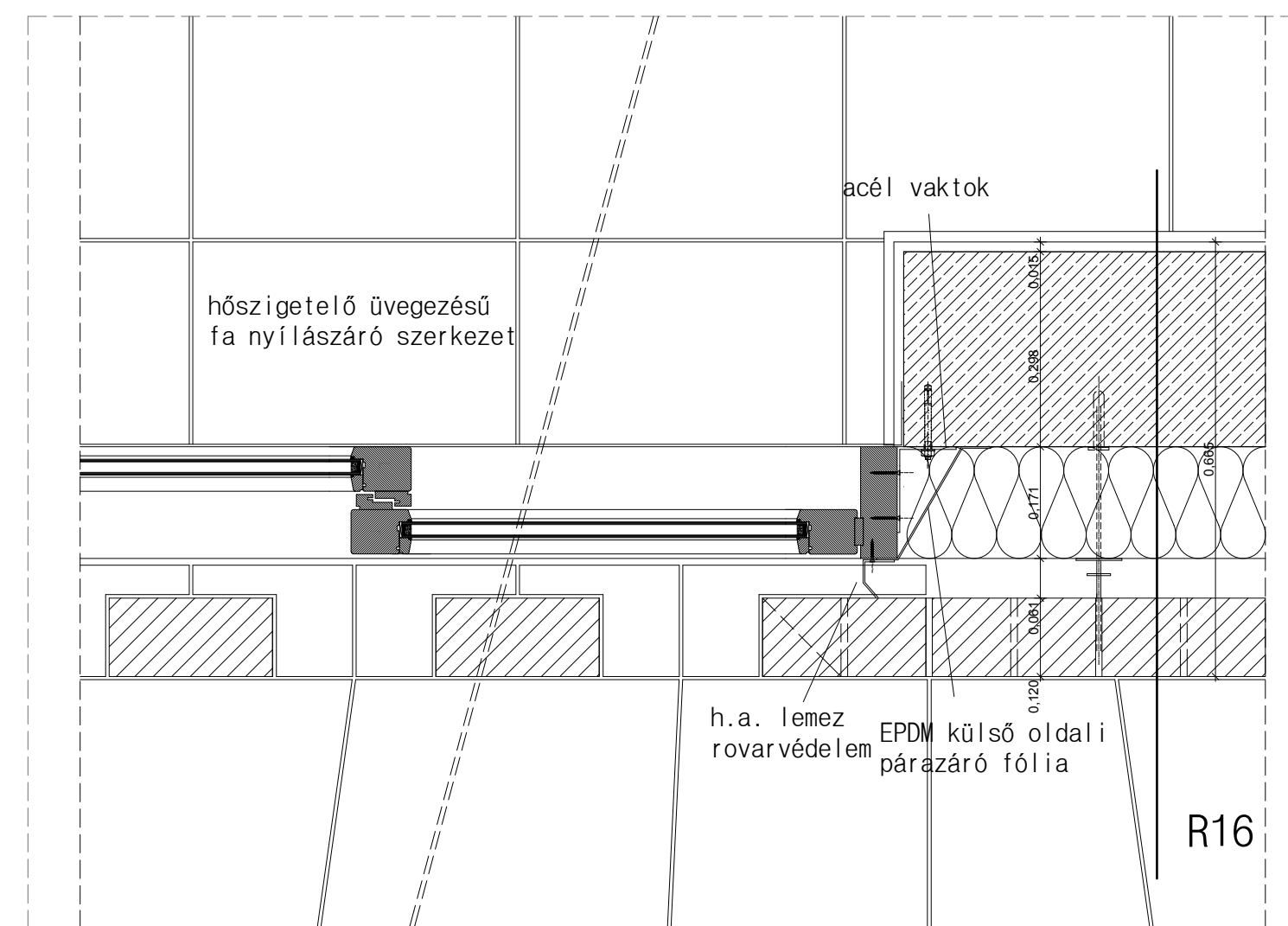
nyílászáró vízszintes metszet
