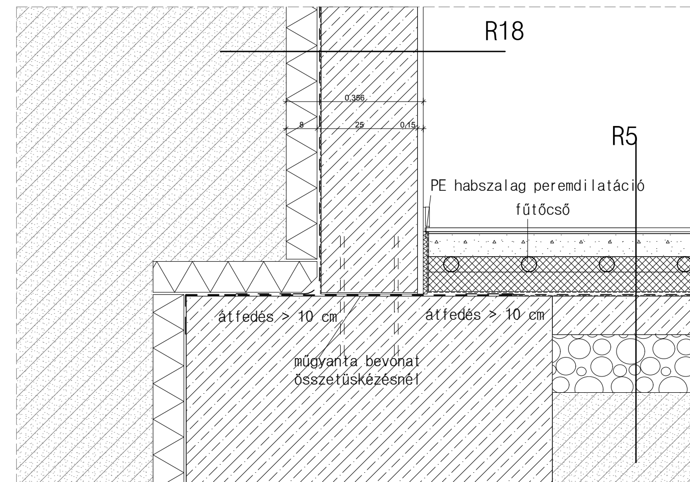
pincefal alapozása
