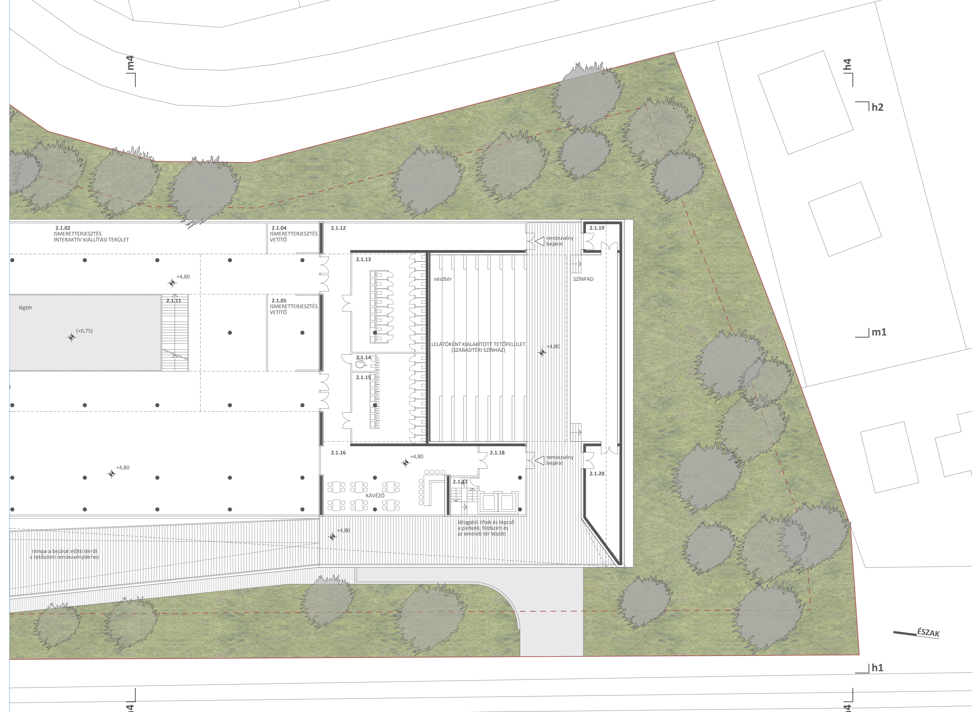
1. EMELETI ALPRAJZ m 1:200
