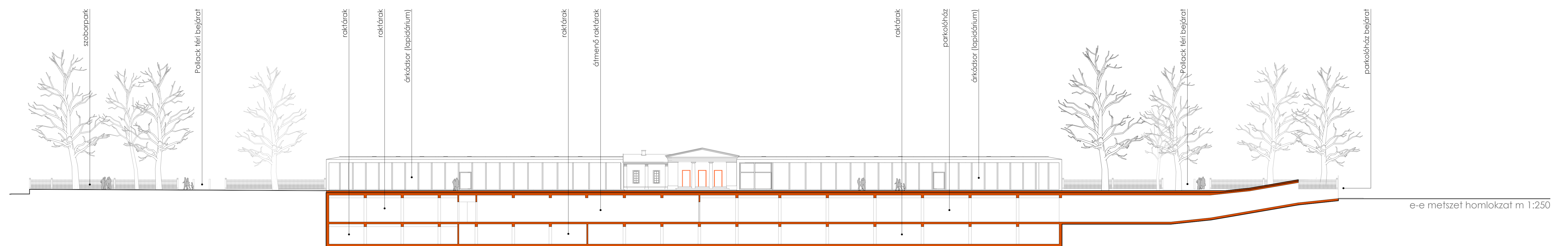
d-d metszet m 1:250
