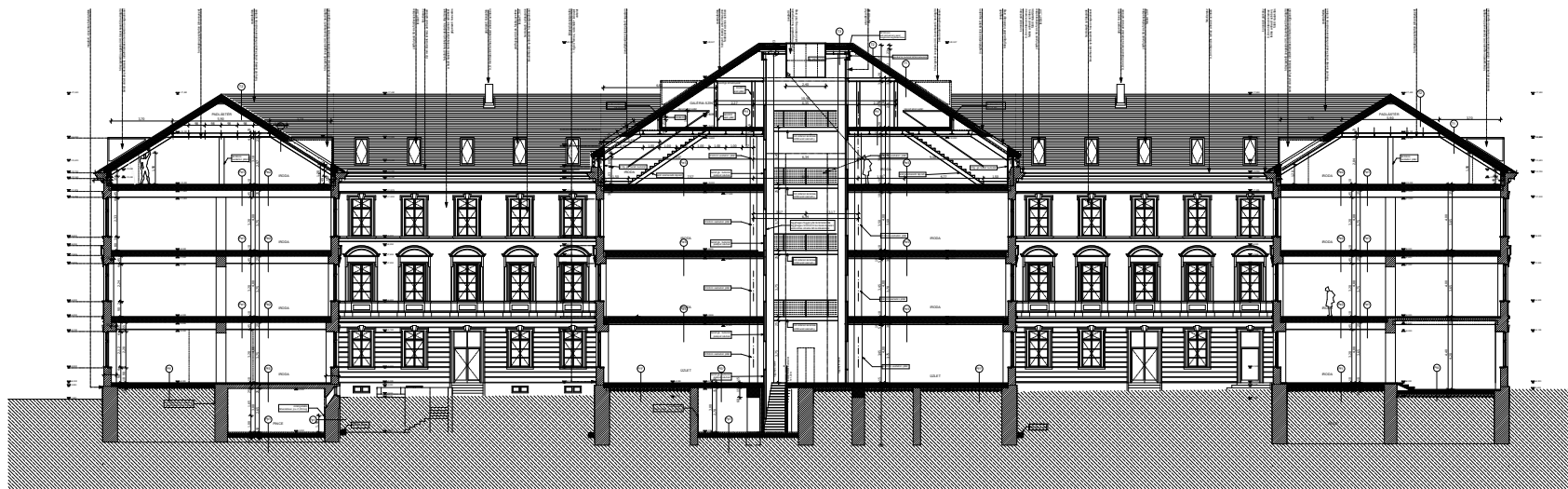
MH1 METSZET
