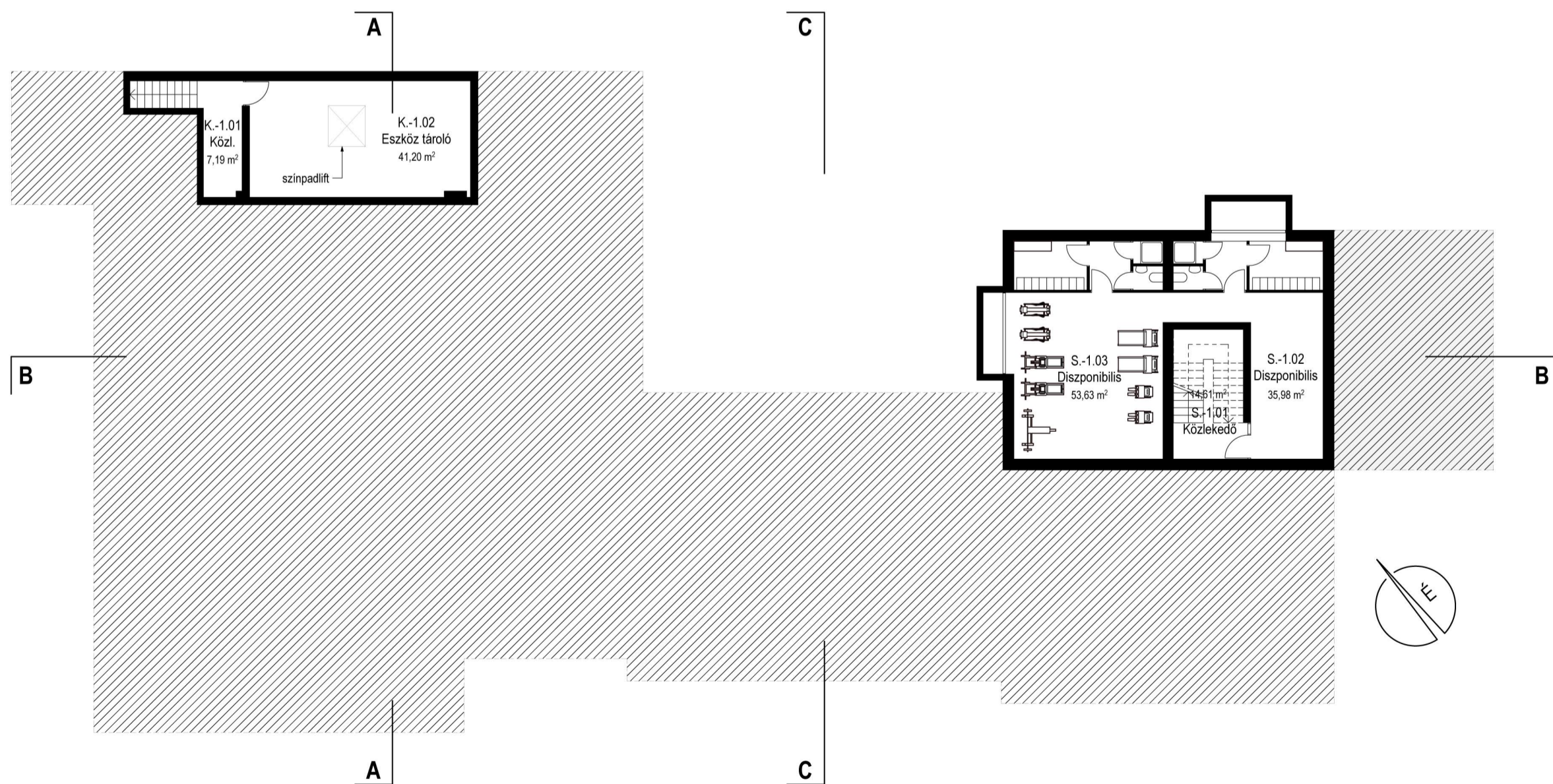
PINCESZINTI ALAPRAJZ M=1:200
