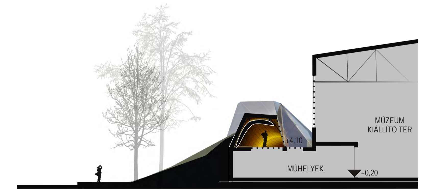
E-E METSZET
