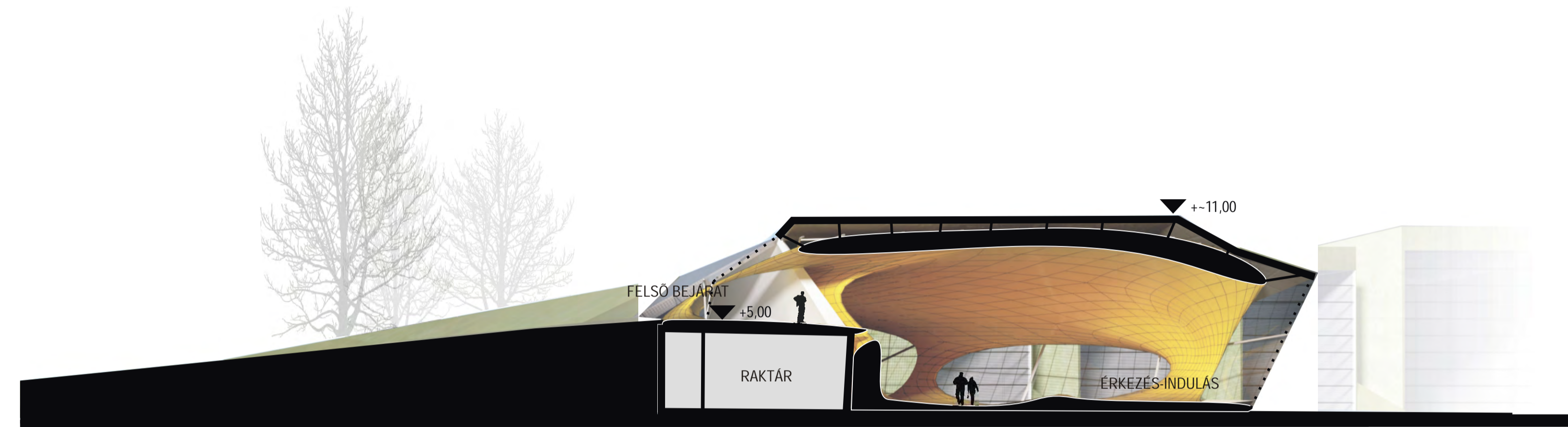
B-B METSZET
