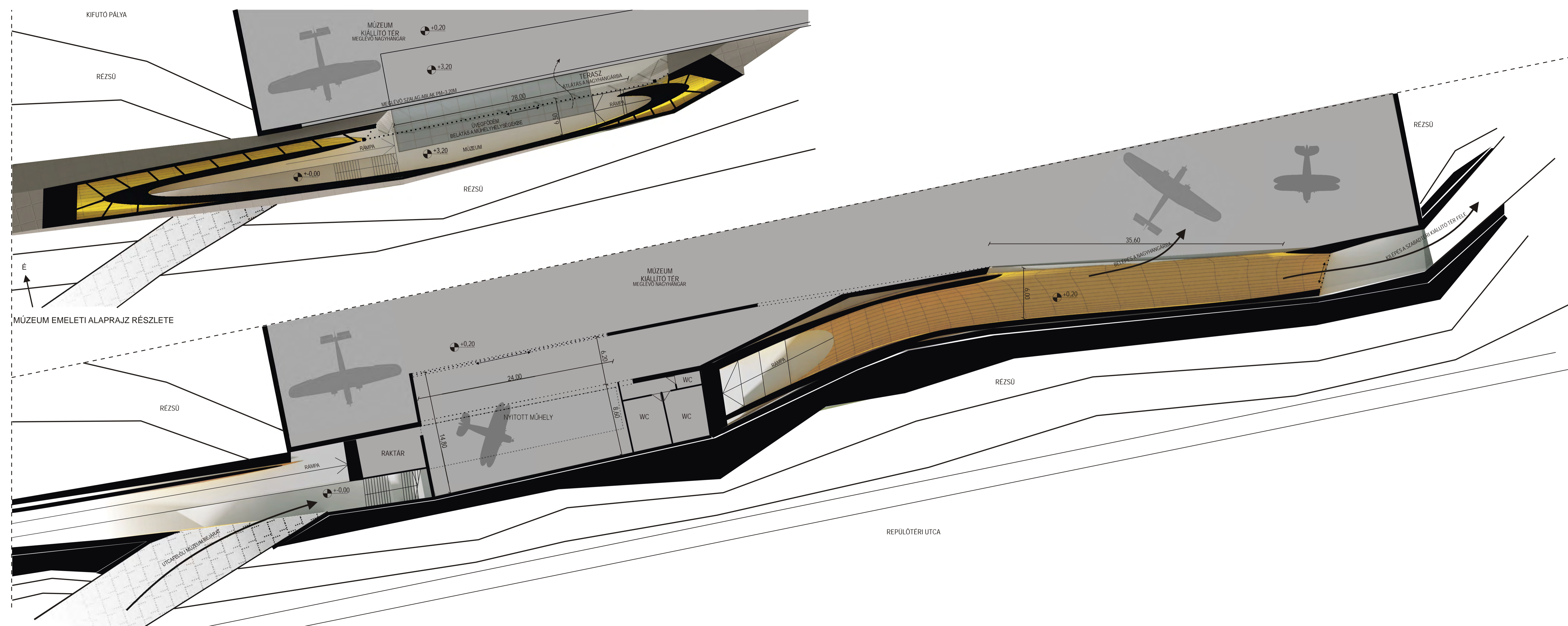
MÚZEUM FÖLDSZINTI ALAPRAJZ RÉSZLETE
