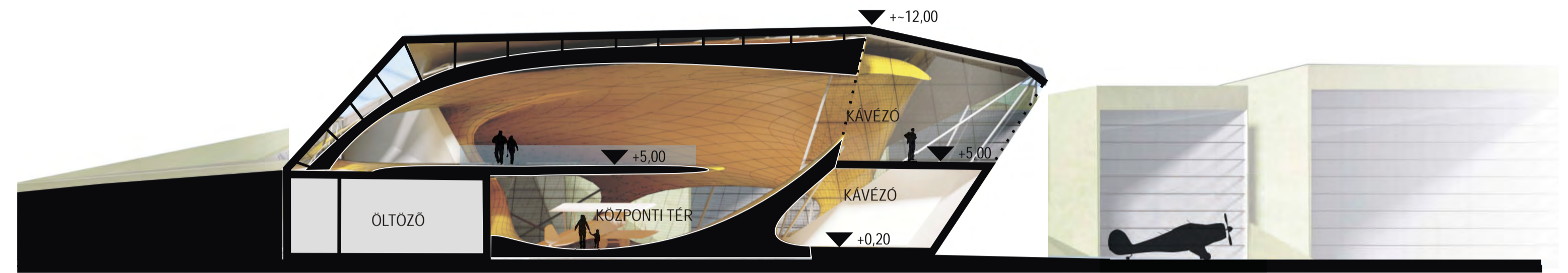
C-C METSZET
