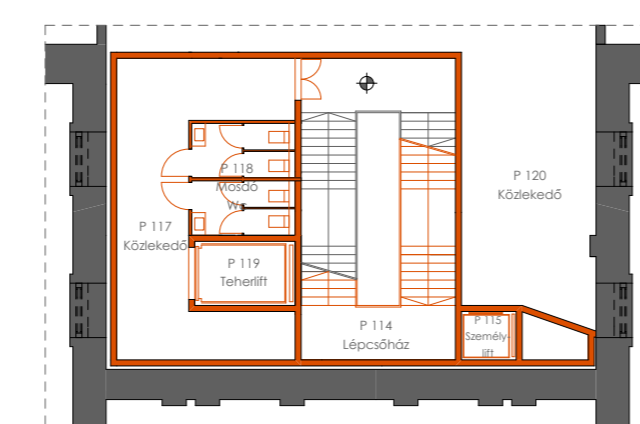
I. - II. félszinti alaprajz m 1:250
