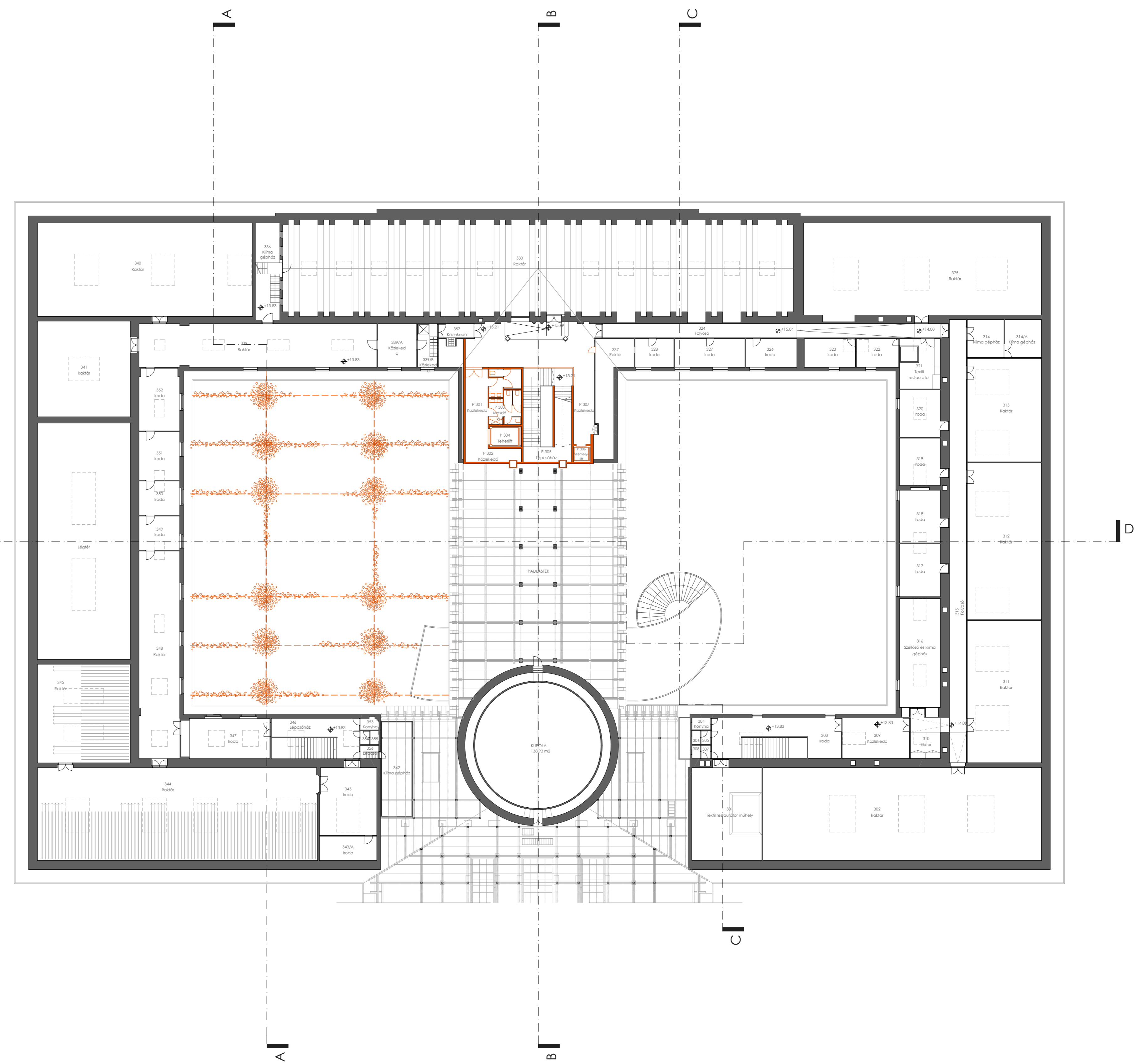
III. szintű alaprajz m 1:250
