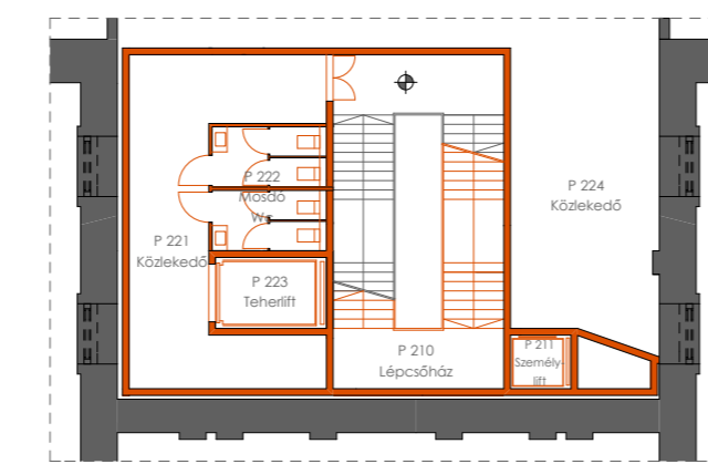
II. - III. félszinti alaprajz m 1:250
