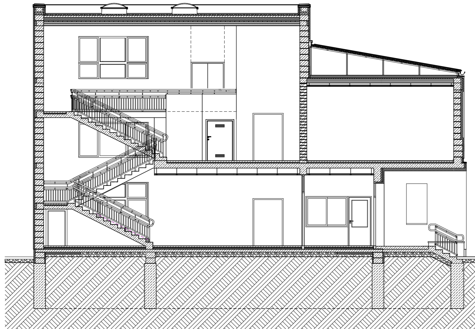
B-B metszet M 1:100
