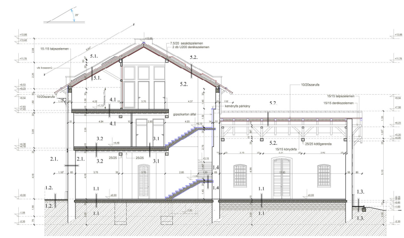
átalakítás utáni a-a metszet m=1:100
