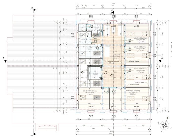
átalakítás utáni 2. emeleti alaprajz m=1:100
