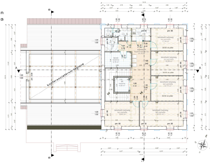
átalakítás utáni 1. emeleti alaprajz m=1:100
