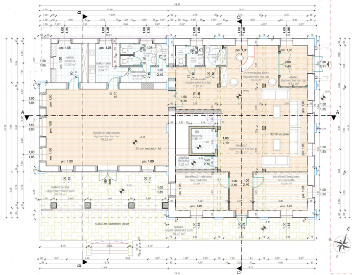
átalakítás után földszinti alapra m=1:100
