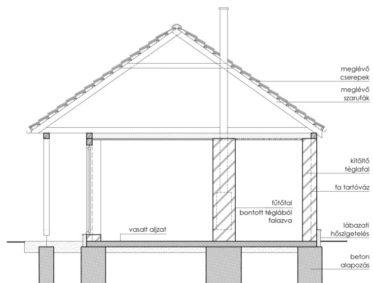
A-A METSZET 1:50
