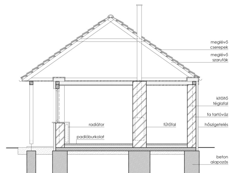
B-B METSZET 1:50
