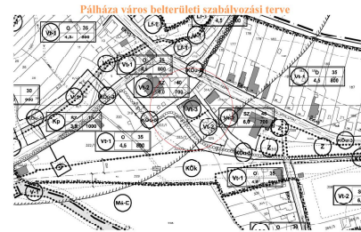
Pálháza város belterületi szabályozási terve
