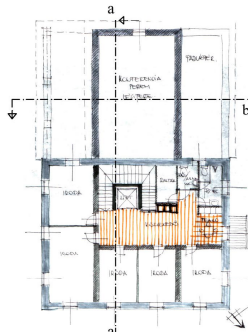
1. emeleti alaprajz m=1:200
