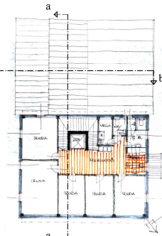
2. emeleti alaprajz m=1:200
