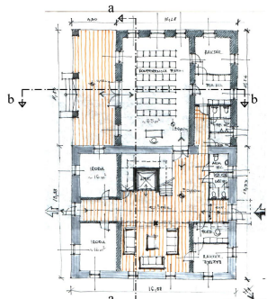
földszinti alaprajz m=1:200
