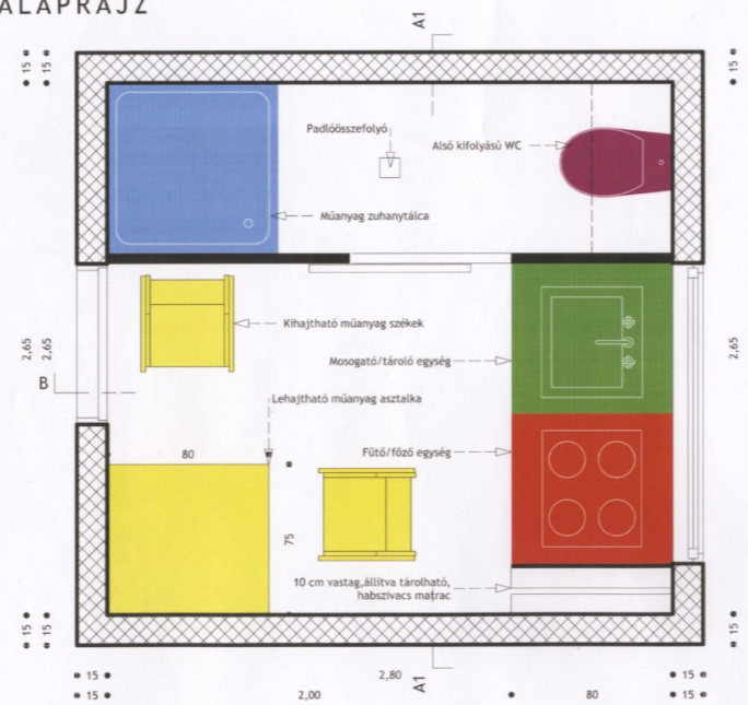
ALAPRAJZ
