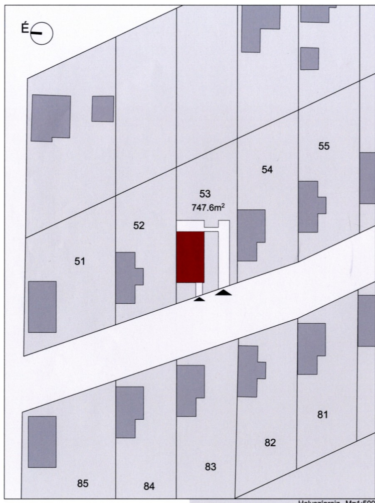
Helyszínrajz M=1:500
