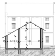
b-b metszet m=1:200
