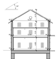
a-a metszet m=1:200
