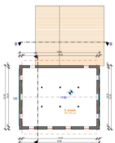
2. emeleti alaprajz m=1:200
