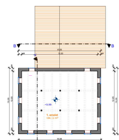
1. emeleti alaprajz m=1:200
