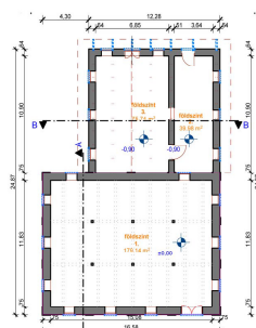
földszinti alaprajz m=1:200
