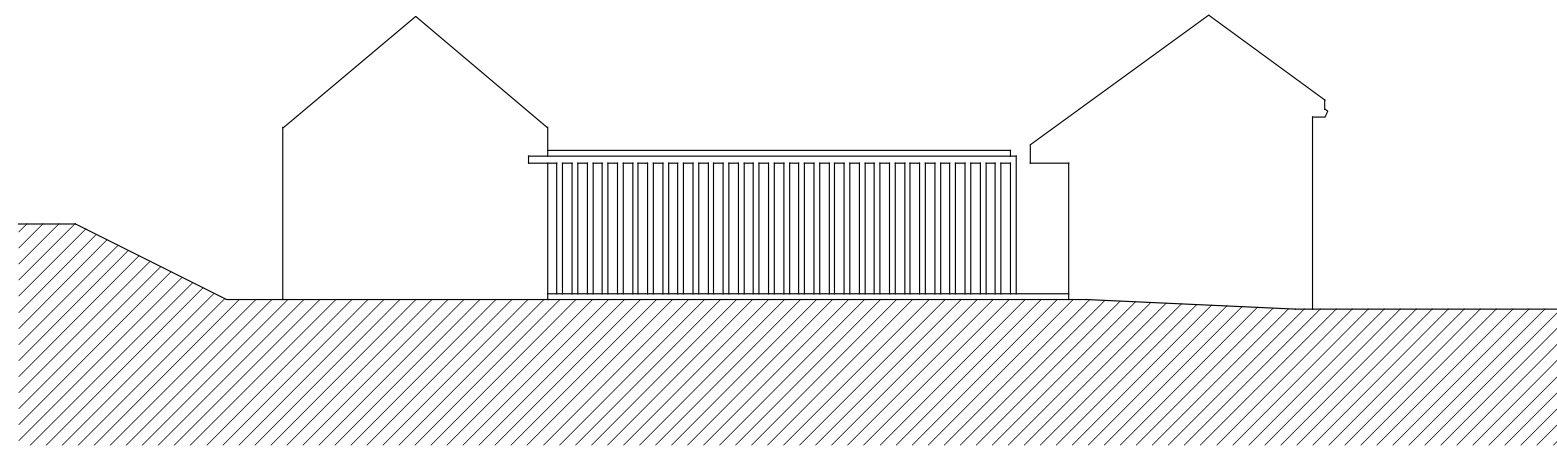
ÉSZAKI HOMLOKZAT
