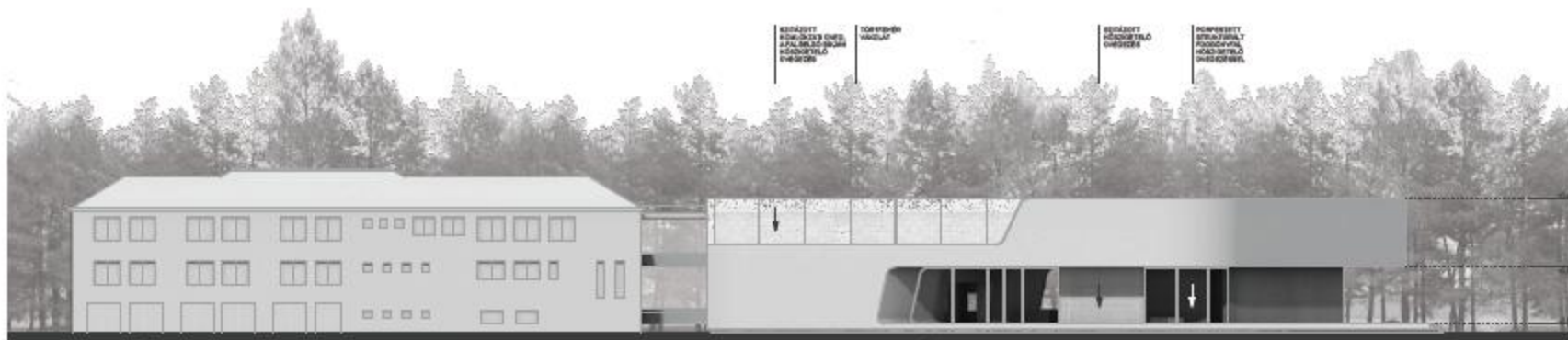
NYUGATI - HORGÁSZ ÚT FELŐLI - HOMLOKZAT M = 1 : 200
