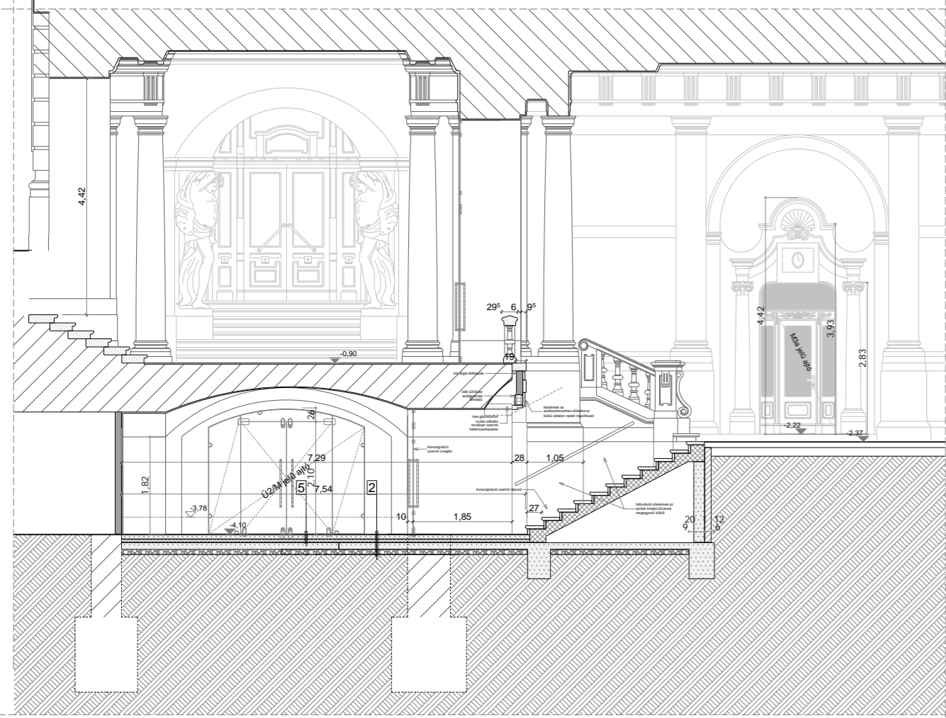
E-E metszet
