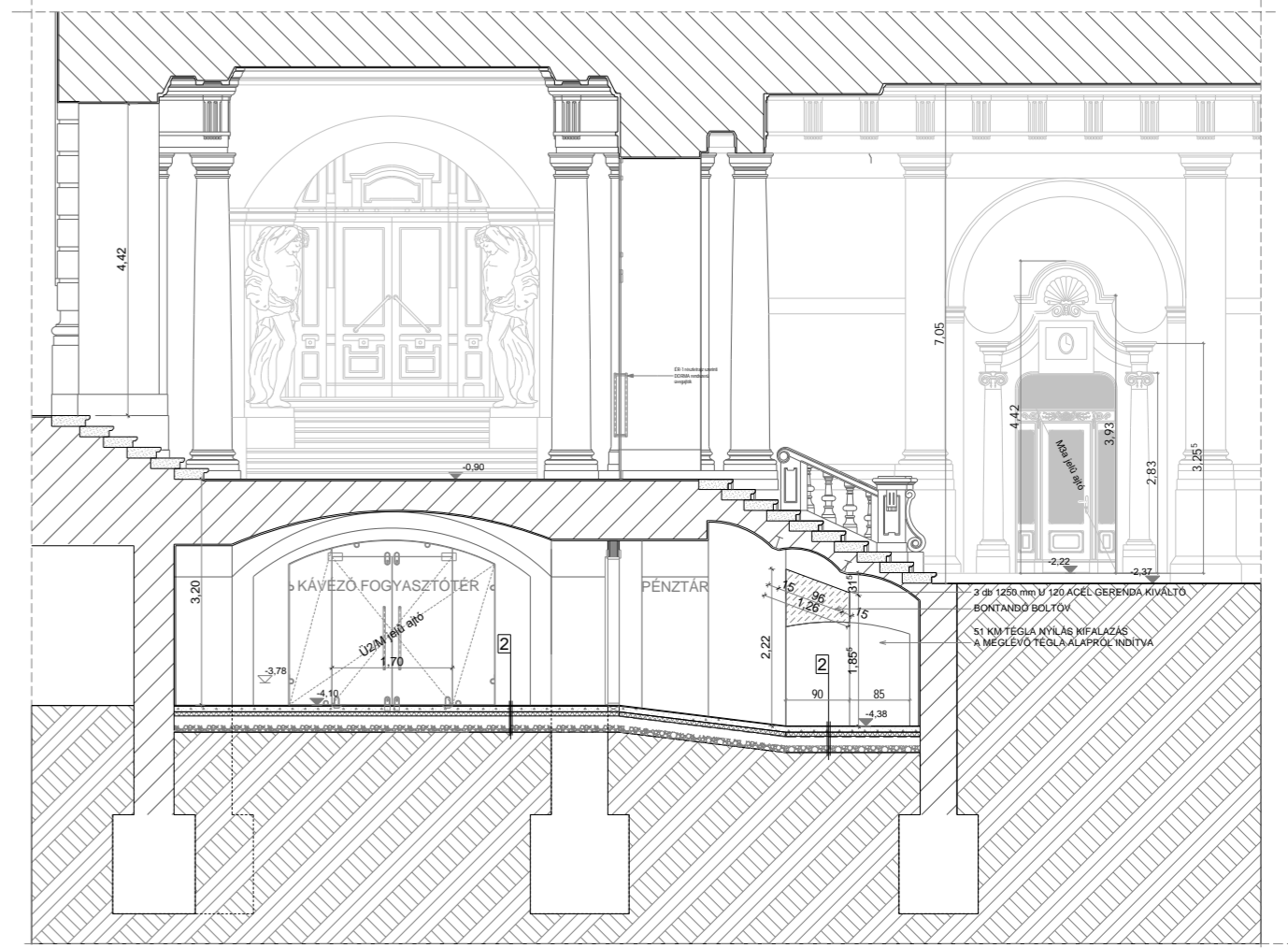
G-G metszet
