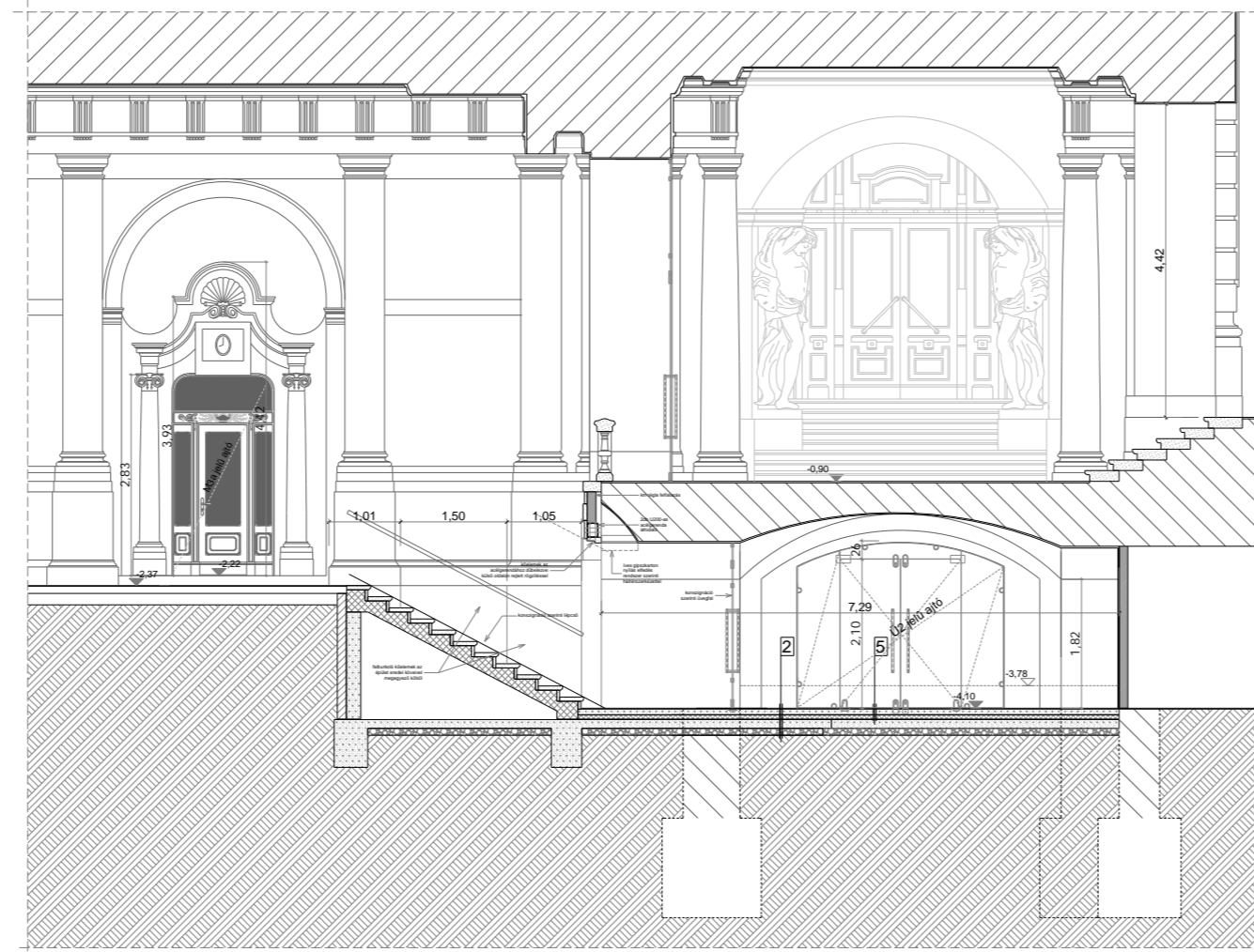
F-F metszet
