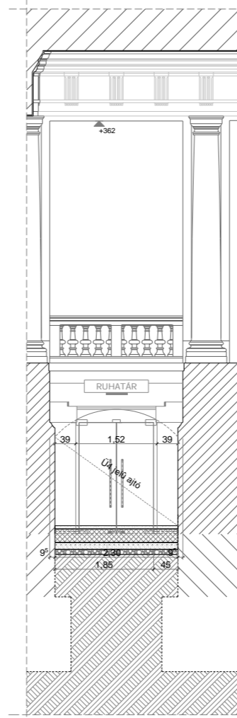
H-H metszet
