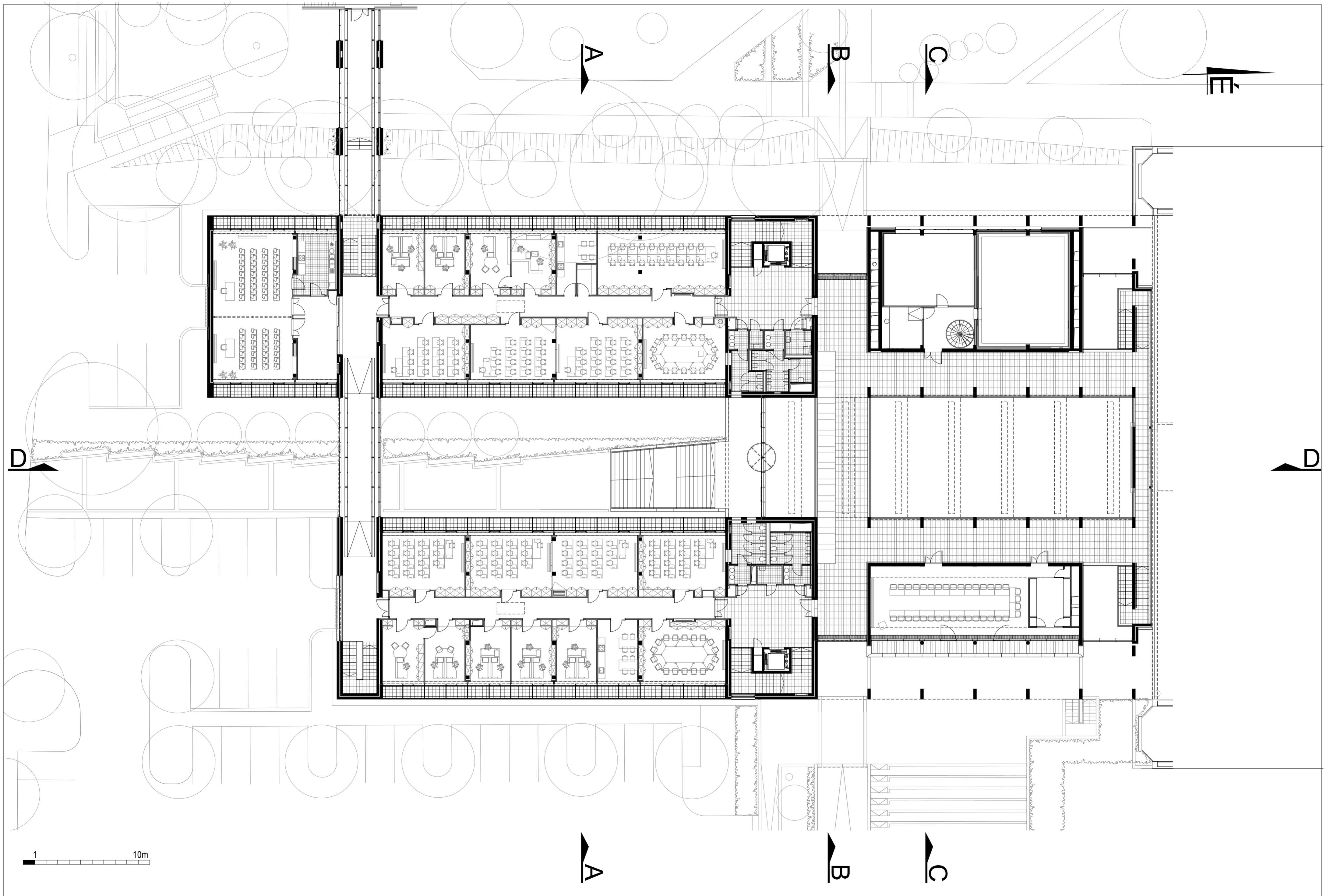
2.EMELETI ALAPRAJZ
