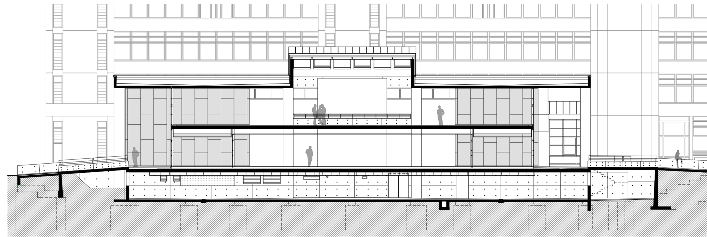
B METSZET
