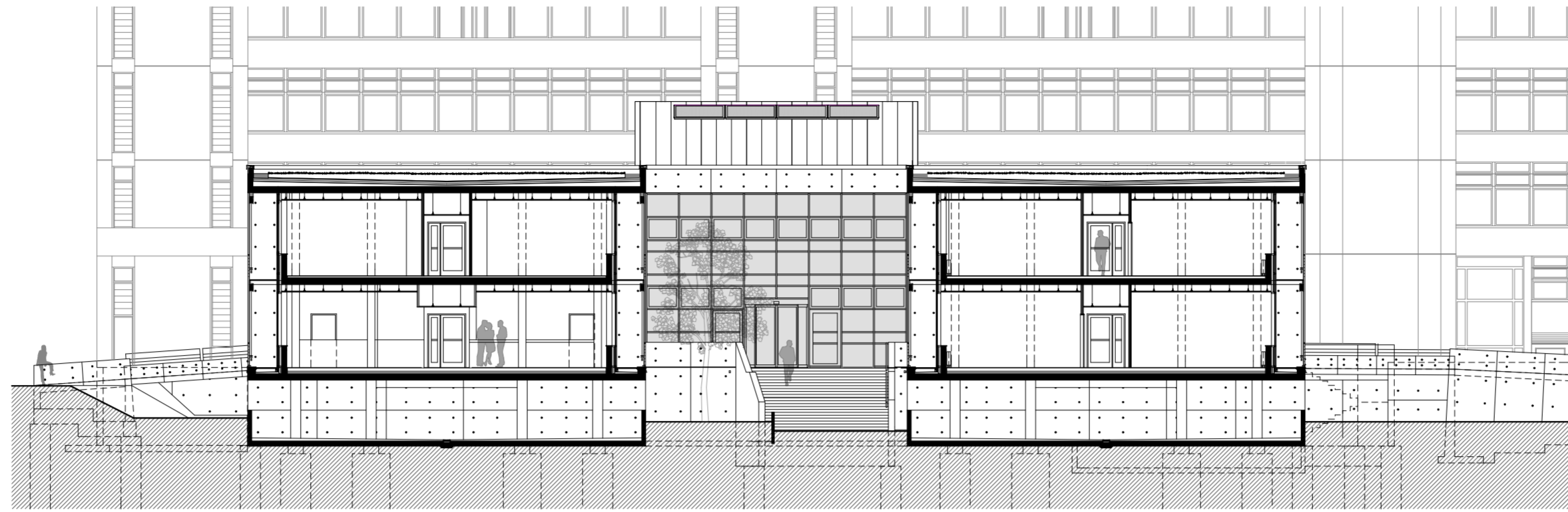
A METSZET
