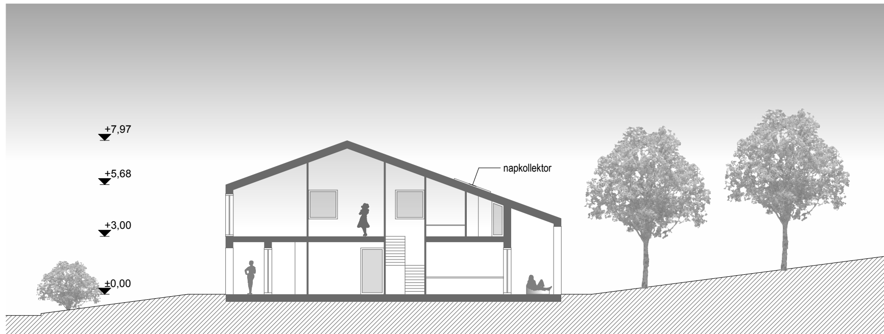
a-a metszet
