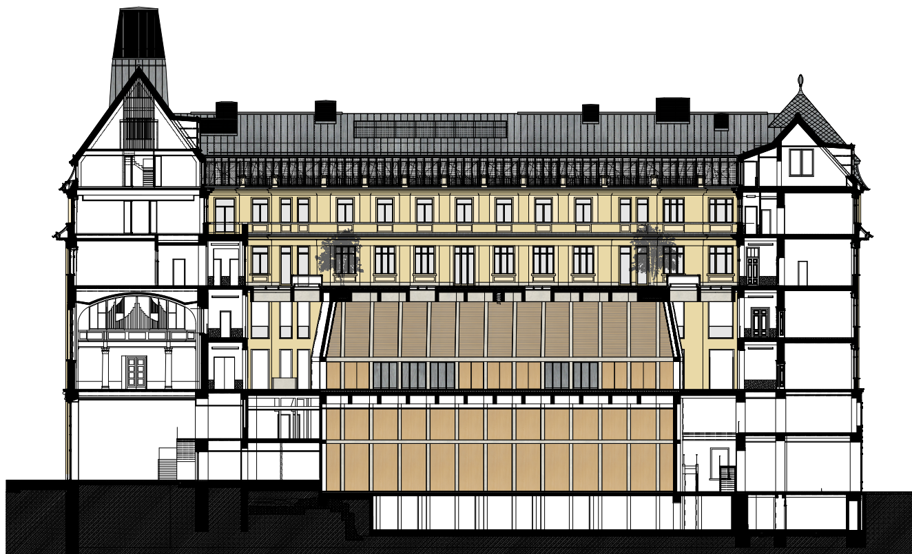
HOSSZMETSZET
