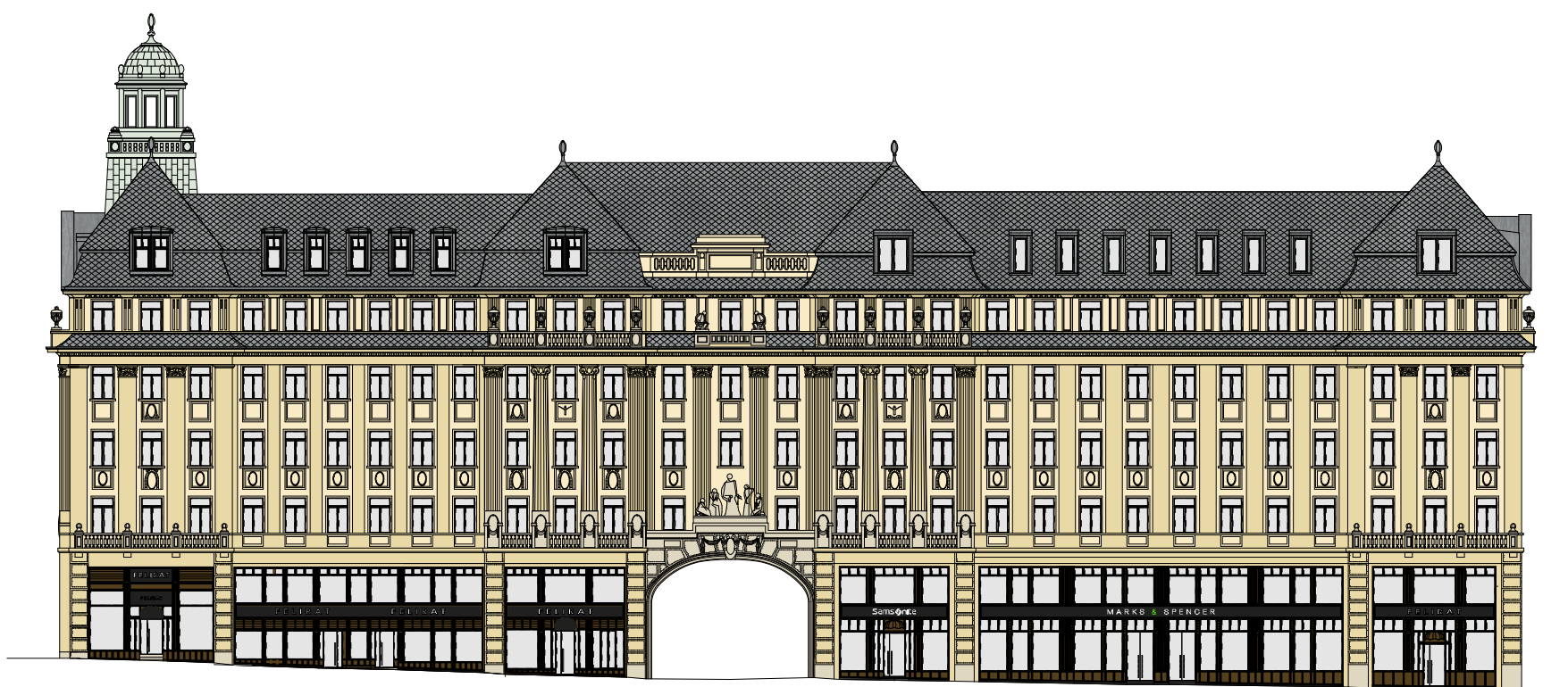
VÁCI UTCAI HOMLOKZAT
