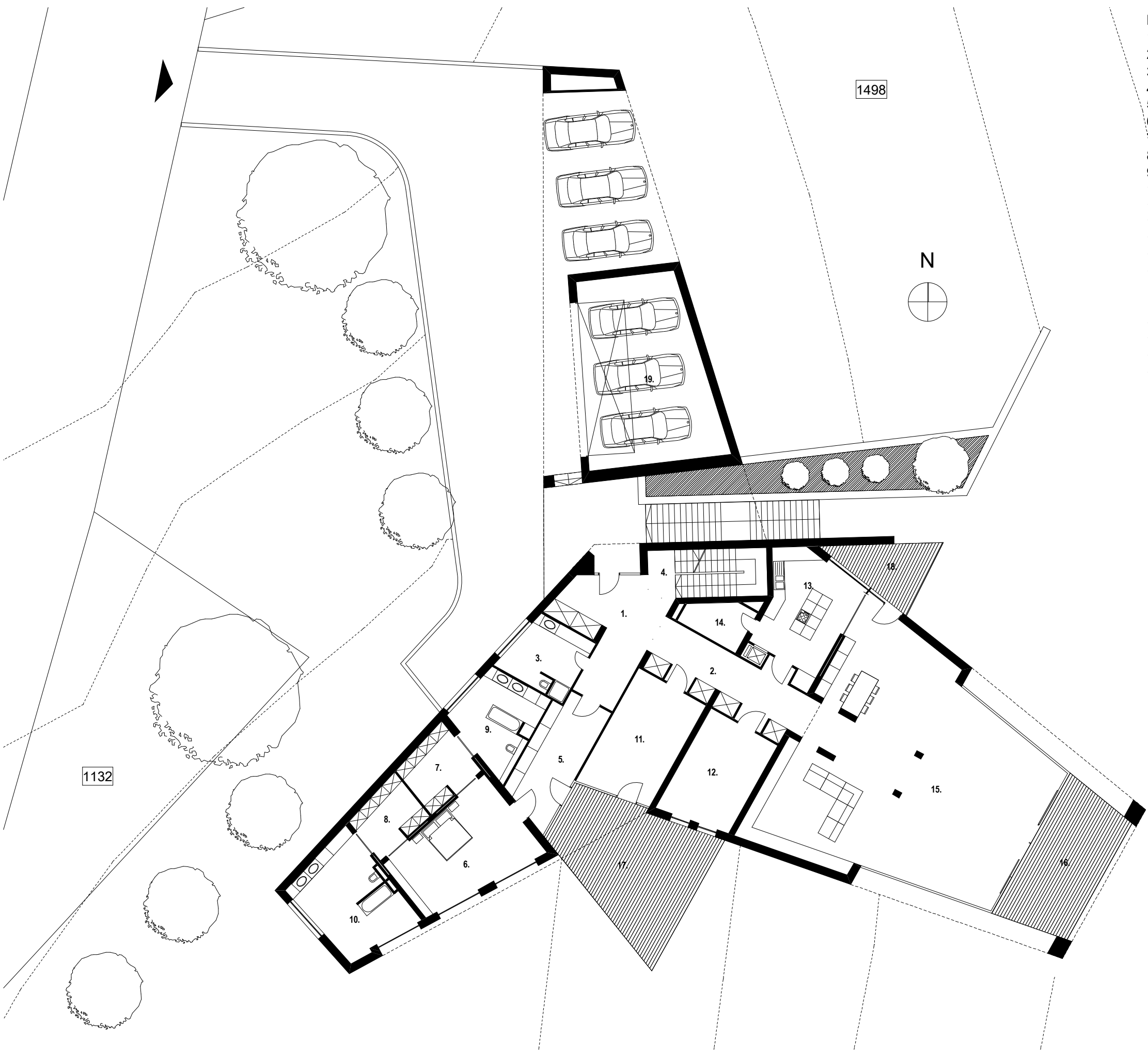
GRUNDRISS EG. - WOHNHAUS EISENBERG - M=1:200 - 1498 Gst.-Nr.
