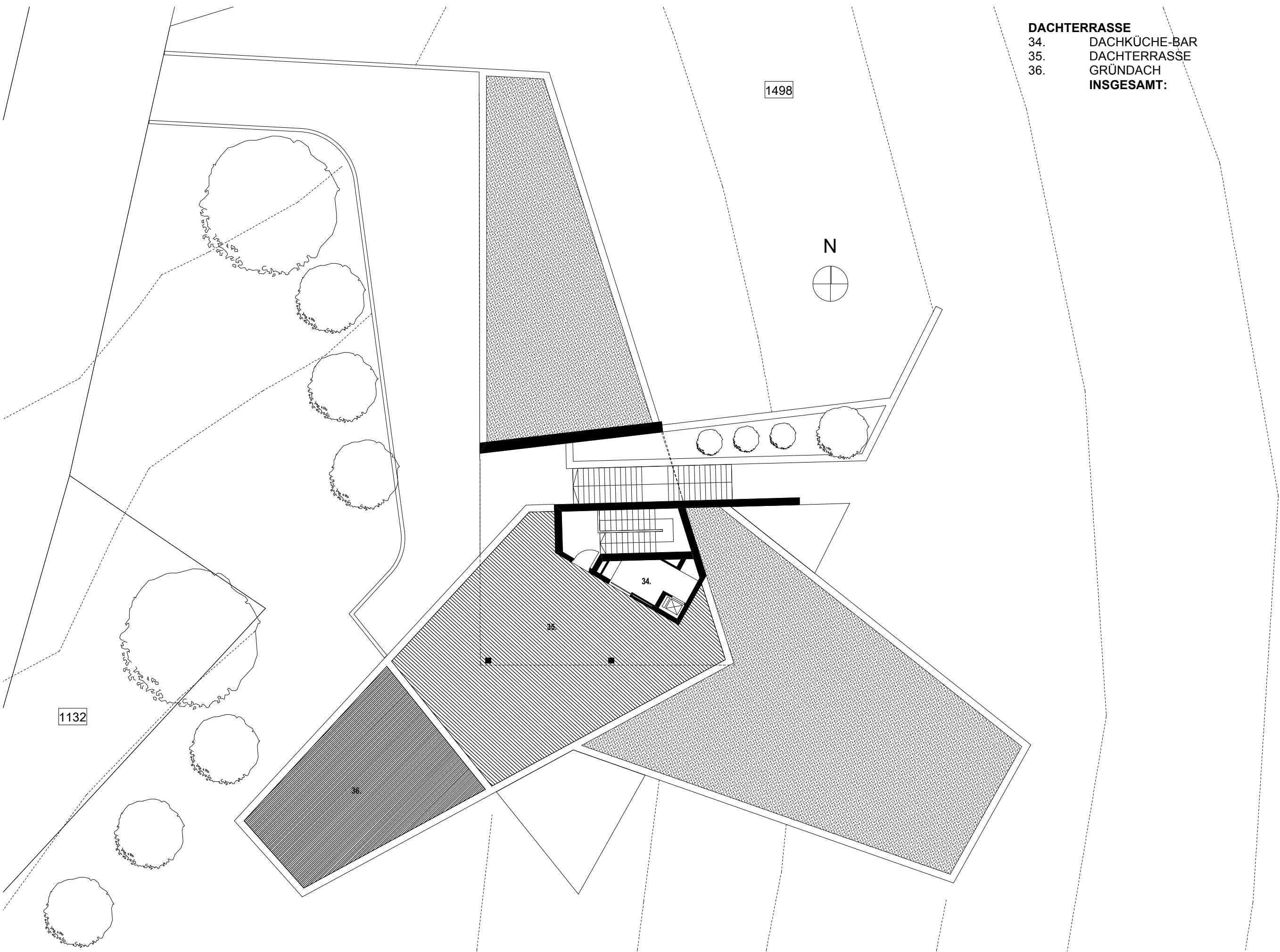
GRUNDRISS OG.-DACHTERRASSE - WOHNHAUS EISENBERG - M=1:200 - 1498 Gst.-Nr.
