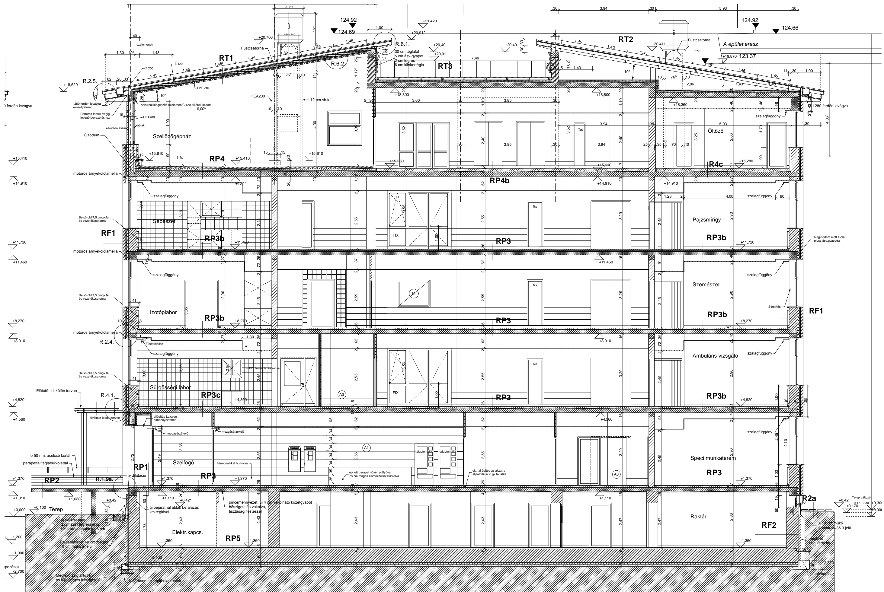
A-1 metszet "R" épület
