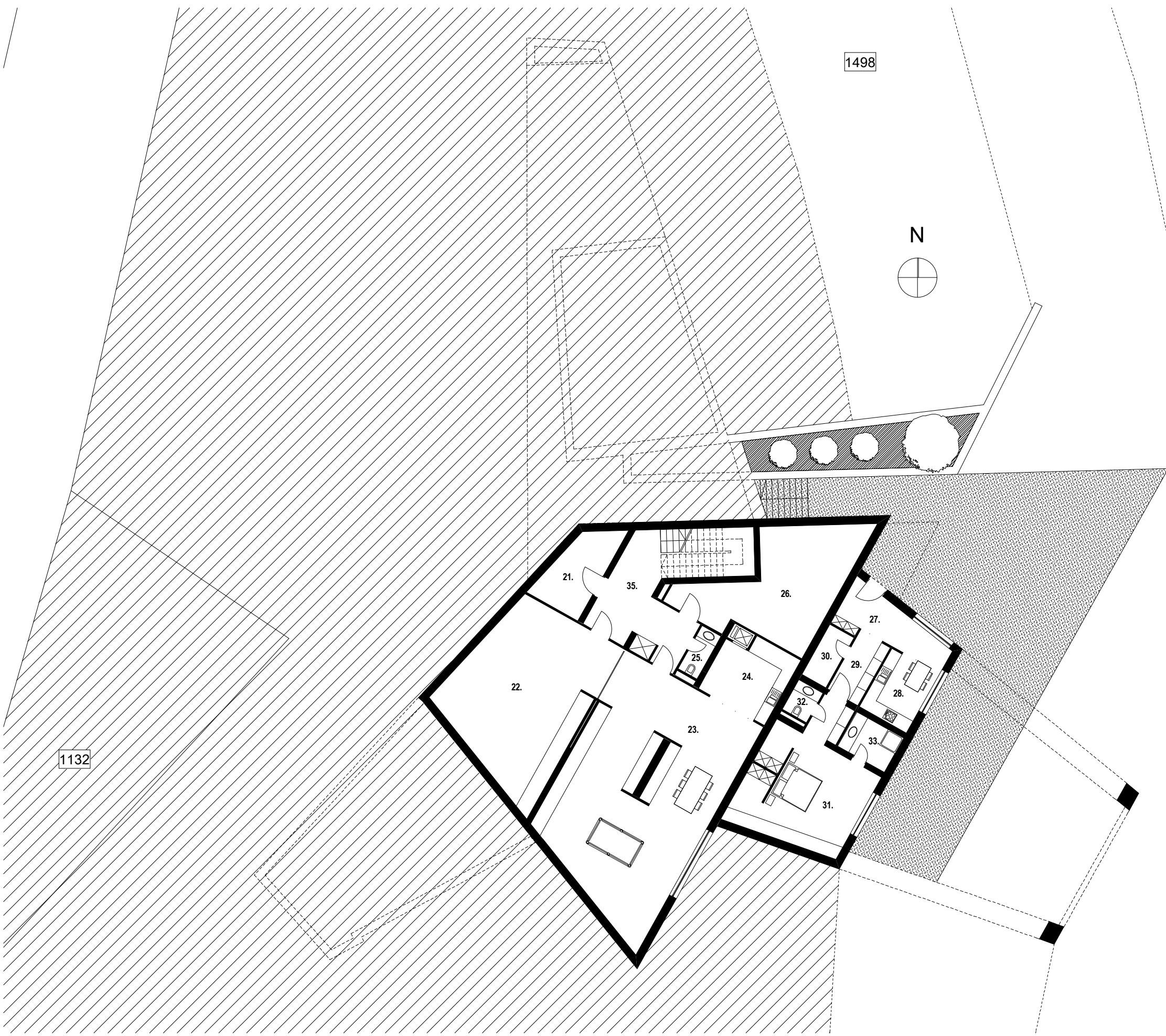
GRUNDRISS UG. - WOHNHAUS EISENBERG - M=1:200 - 1498 Gst.-Nr.
