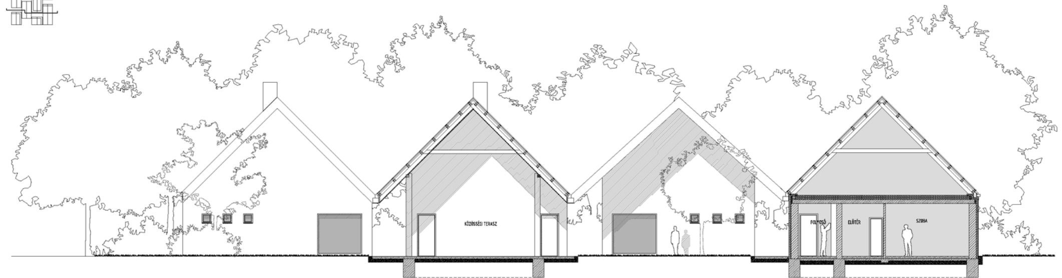
BB METSZET
