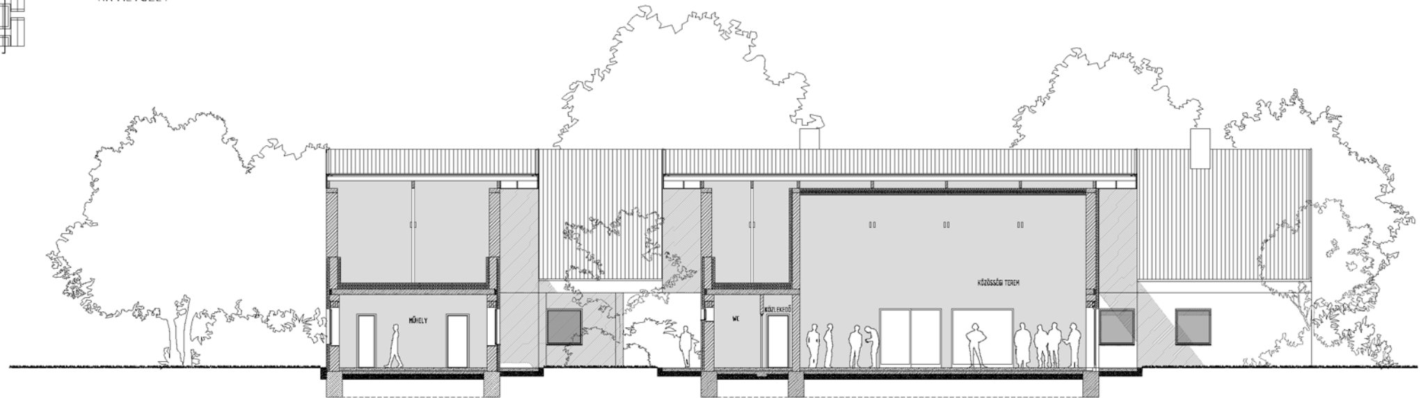
KK METSZET
