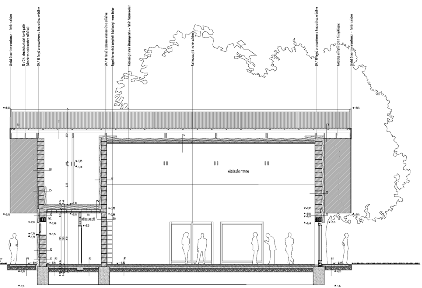
NN METSZET
