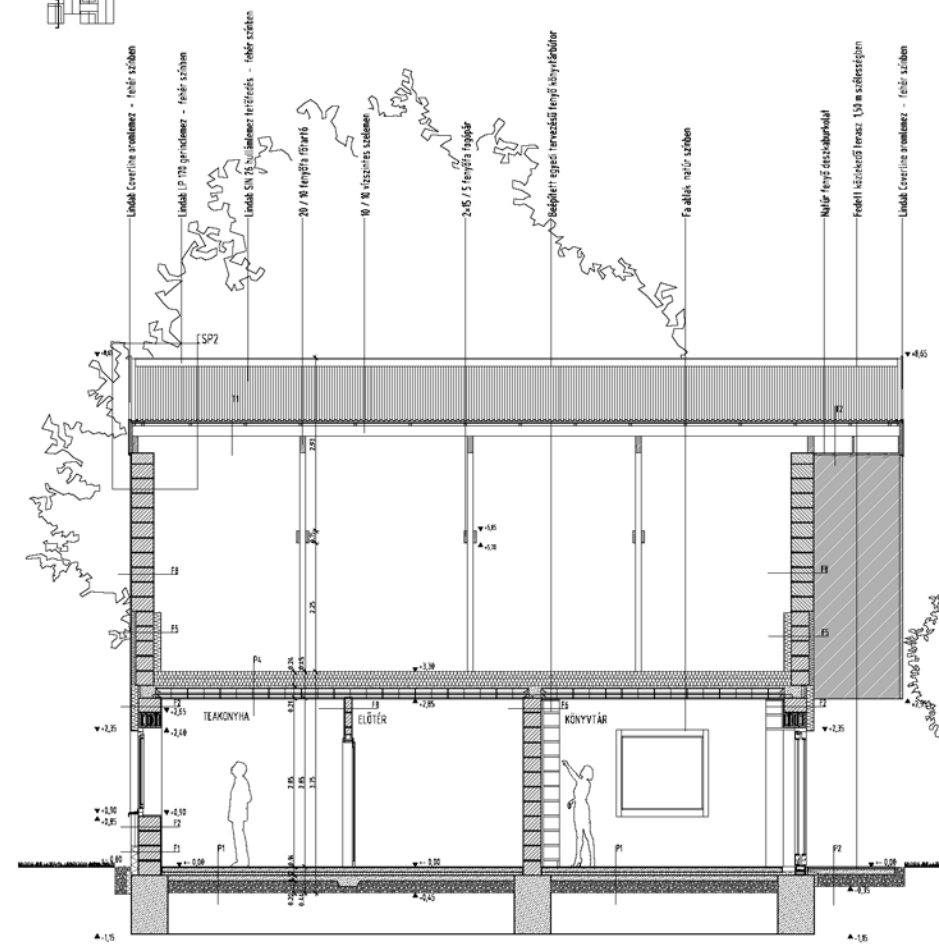
MM METSZET
