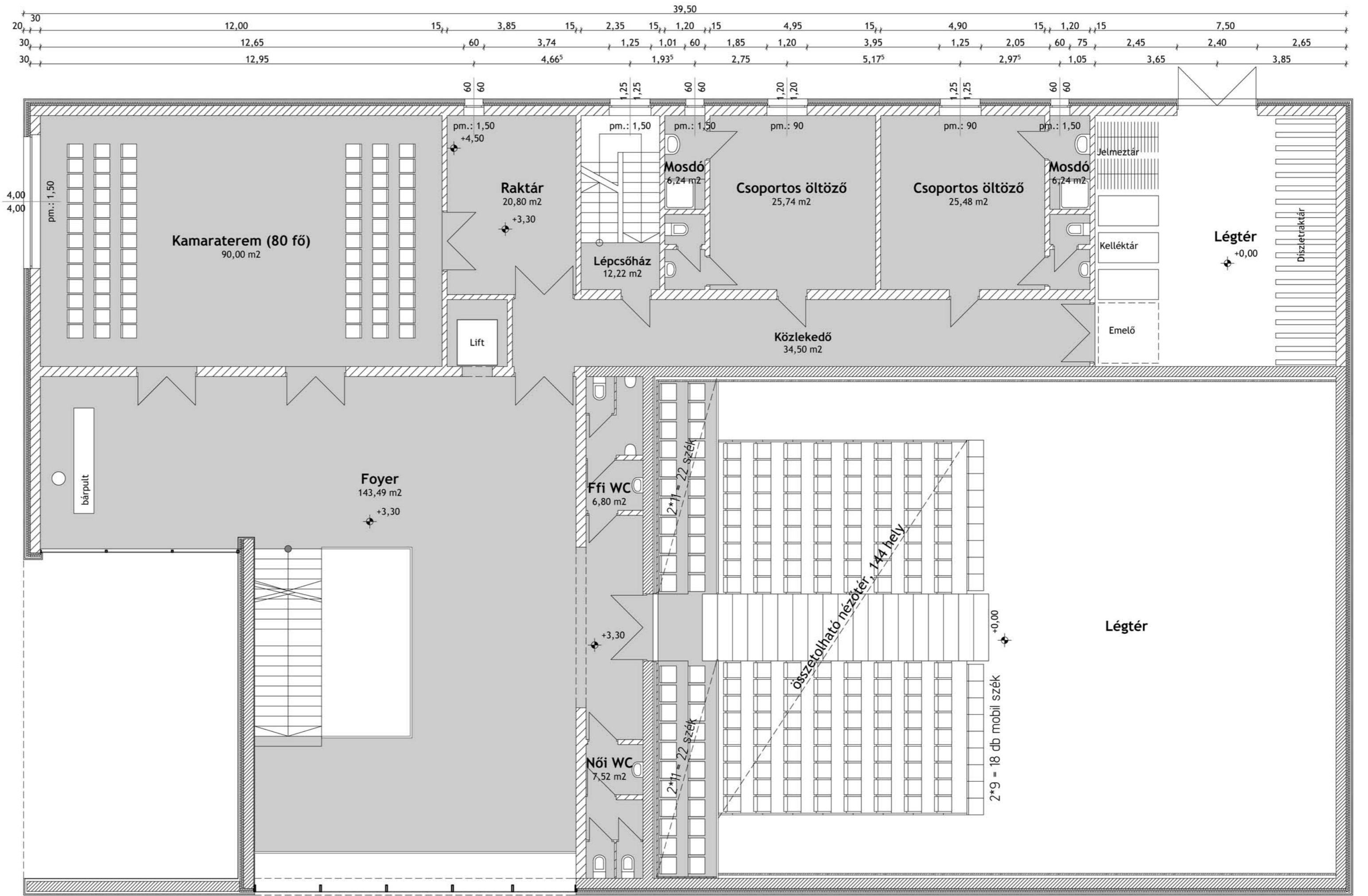
Összetolható nézőtér
