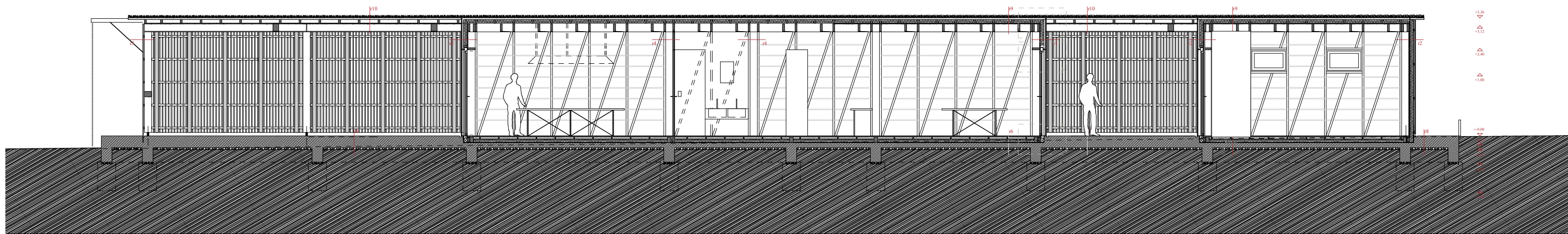
a-a 1:50
