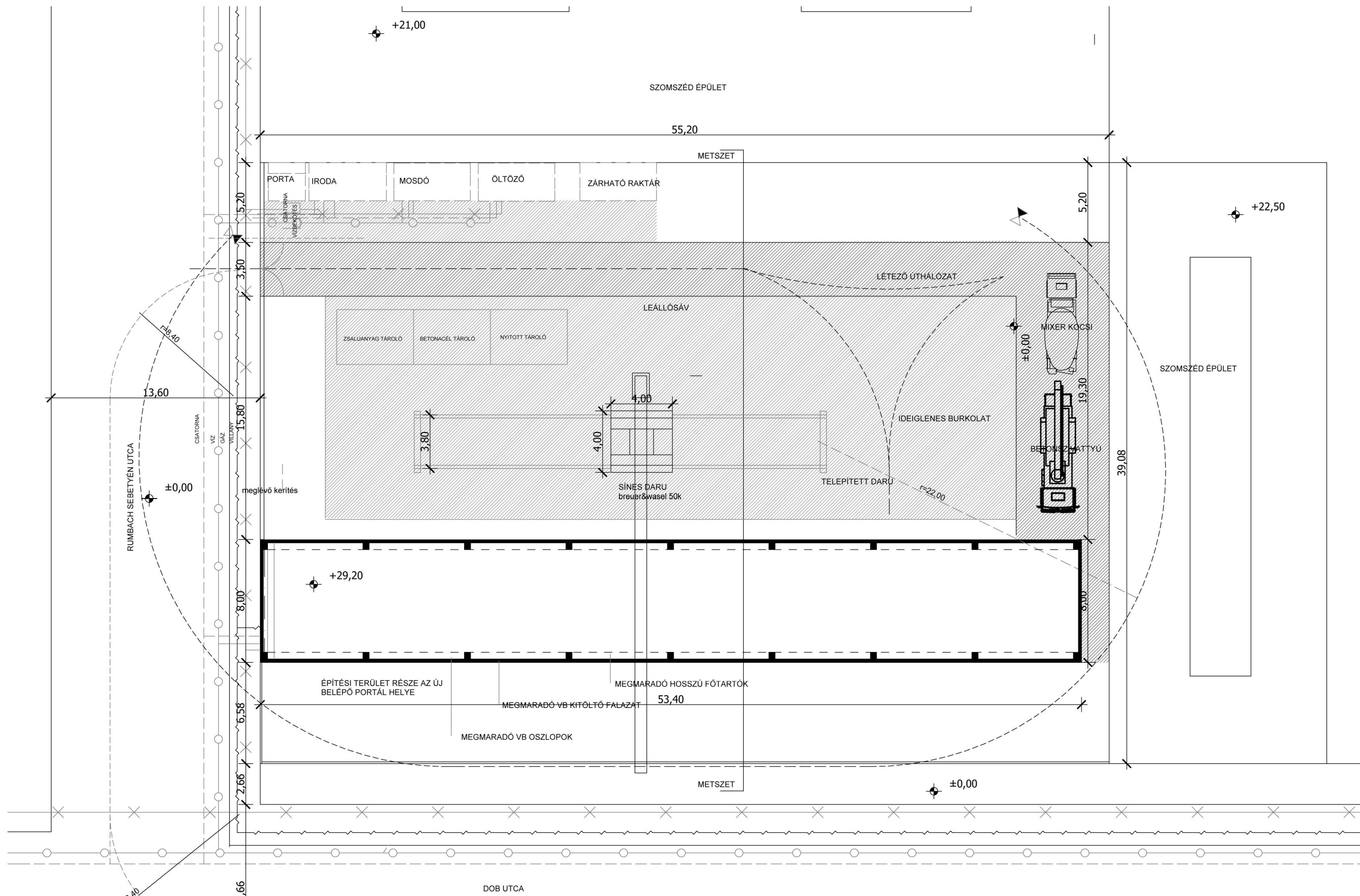
organizációs alaprajz 1:250
