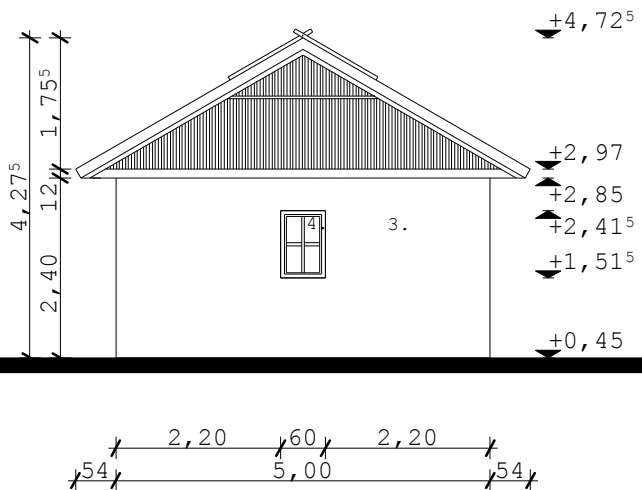
HOMLOKZAT M 1:100
