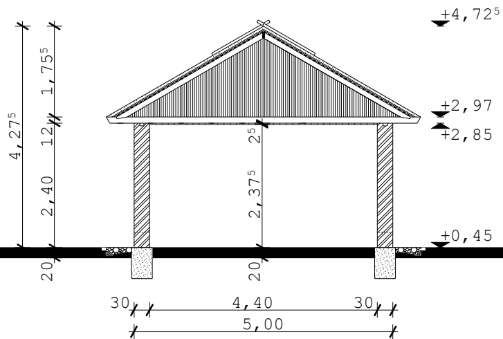
METSZET M 1:100
