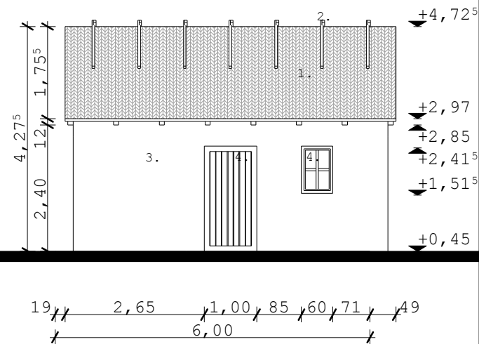
HOMLOKZAT M 1:100
