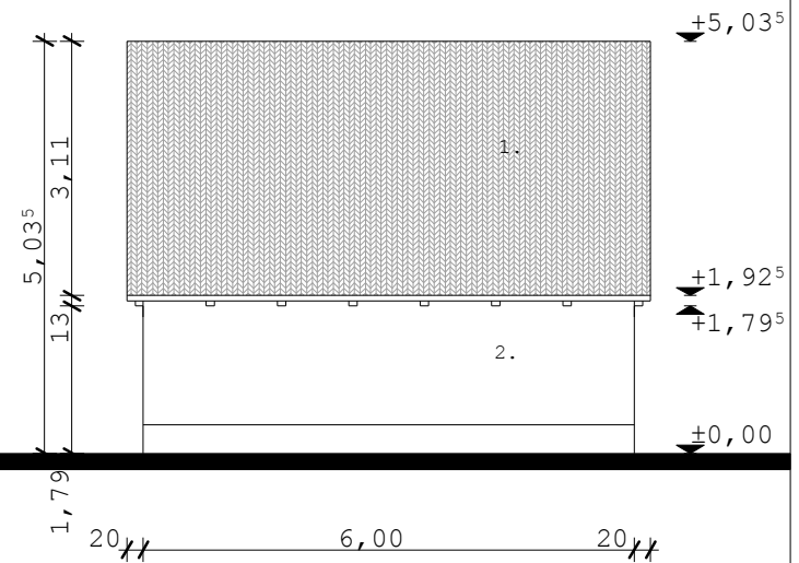
HOMLOKZAT M 1:100
