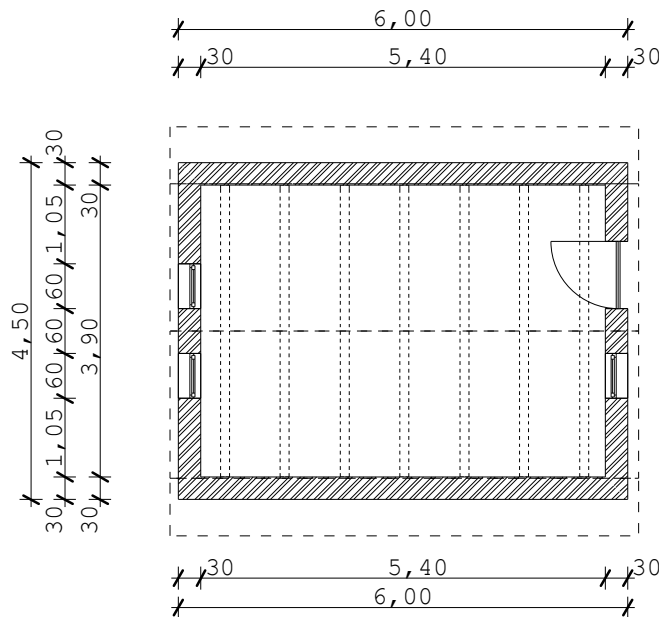
ALAPRAJZ M 1:100
