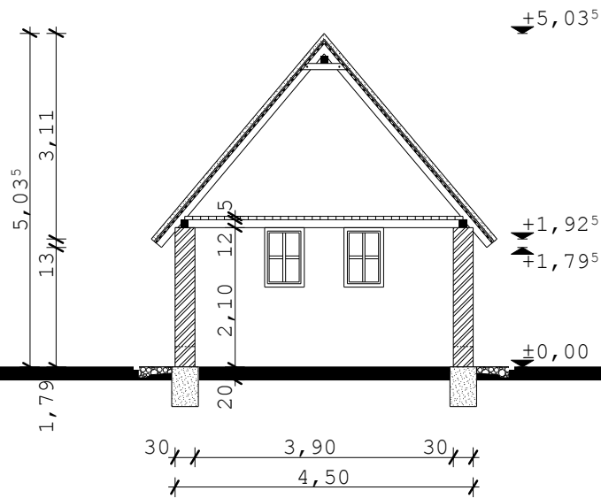
METSZET M 1:100
