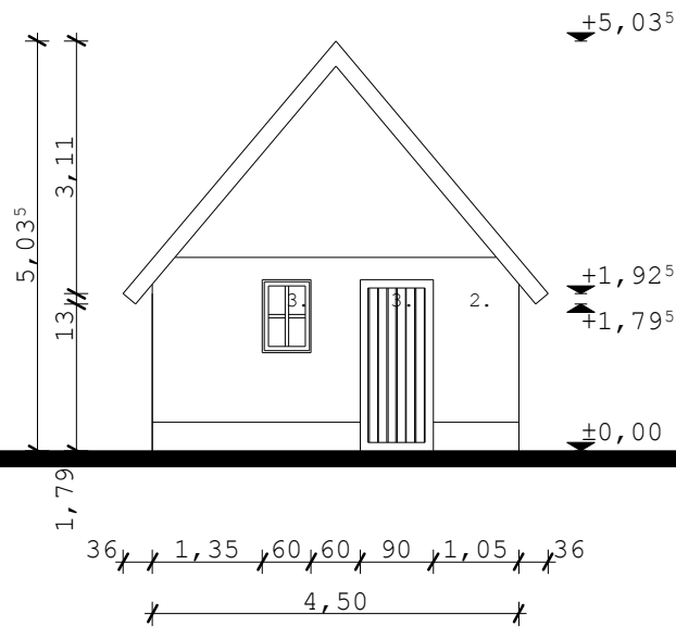
HOMLOKZAT M 1:100
