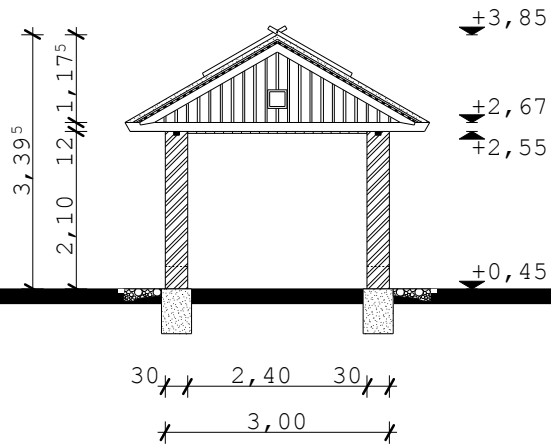
METSZET M 1:100
