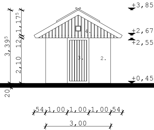
HOMLOKZAT M 1:100
