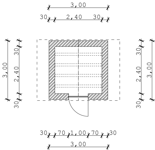
ALAPRAJZ M 1:100
