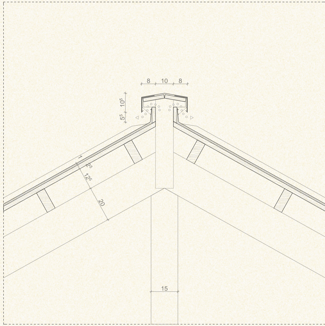
lepárló épületének gerincszellőzése
