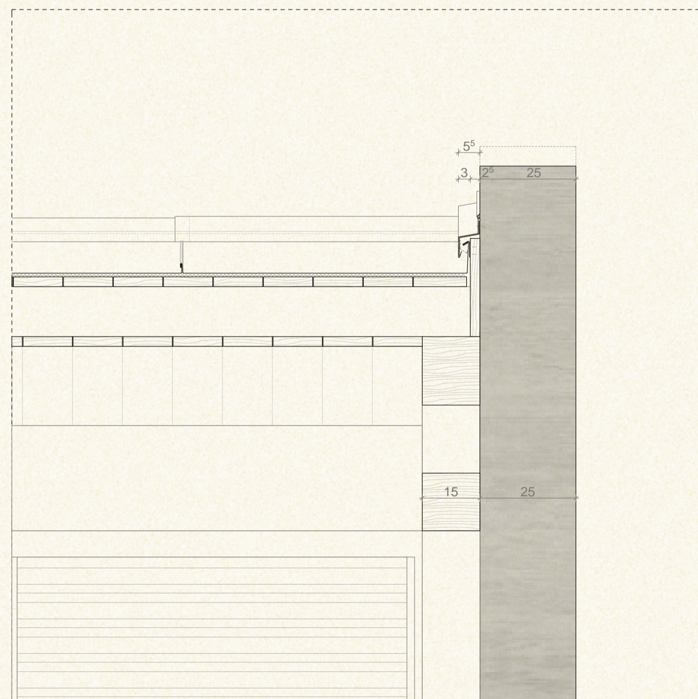
erjesztő épületének orom kialakítása
