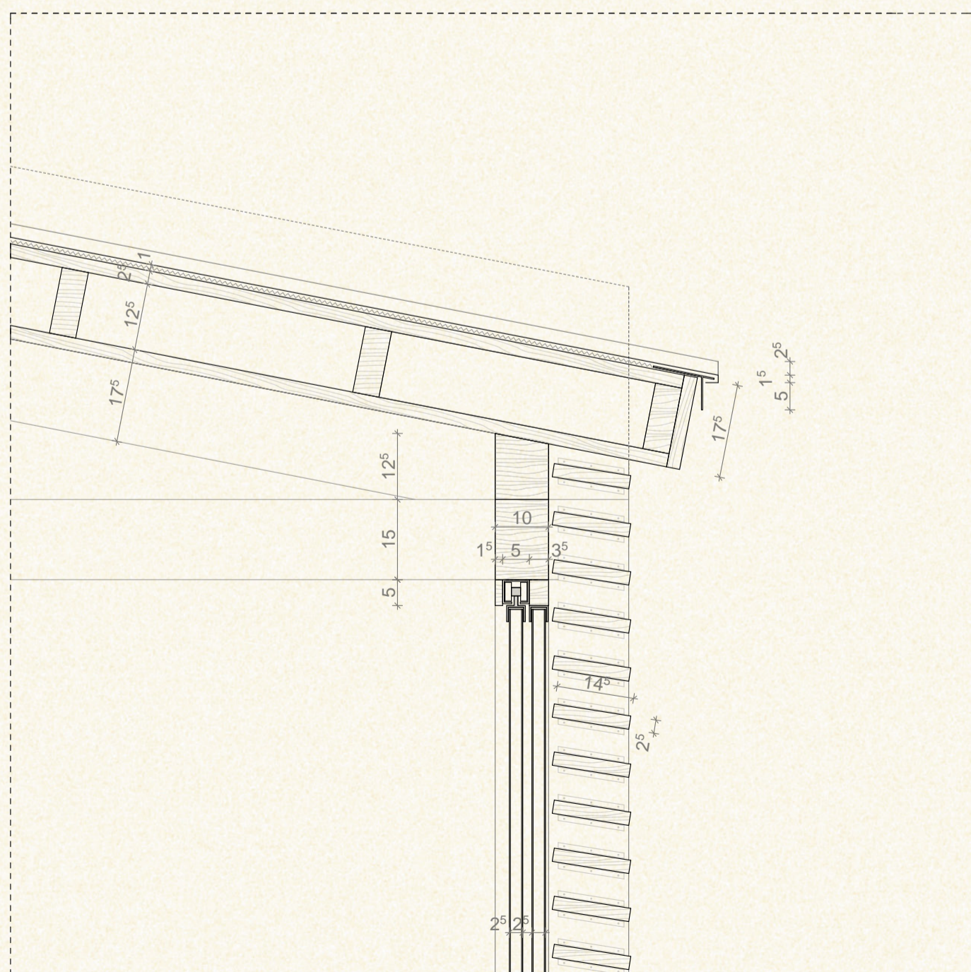
erjesztő épületének ereszképzése
