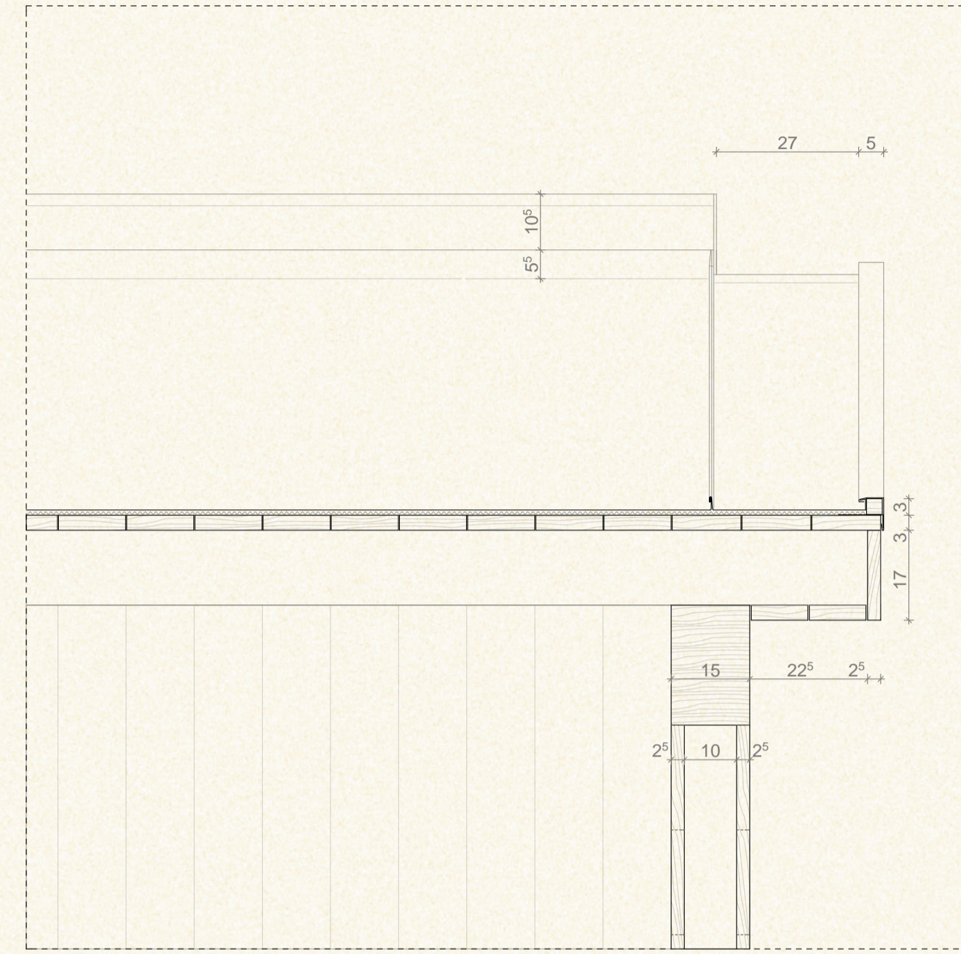
lepárló épületének oromszegély képzése
