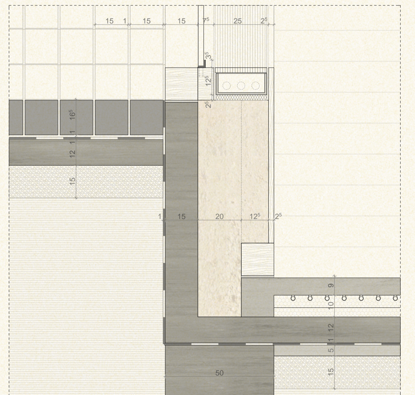
tornác lépcső és a beltér kapcsolata
