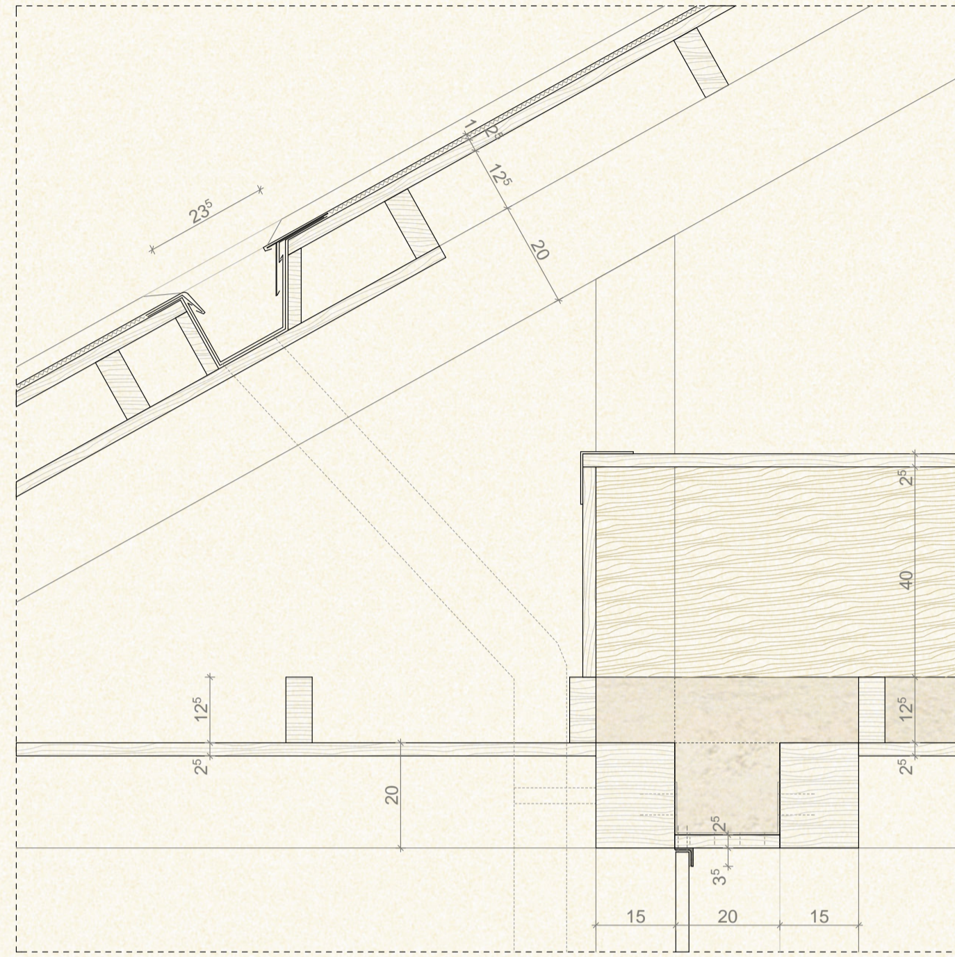
lepárló épületének tornácoldali csatorna- illetve fix ablak kialakítása
