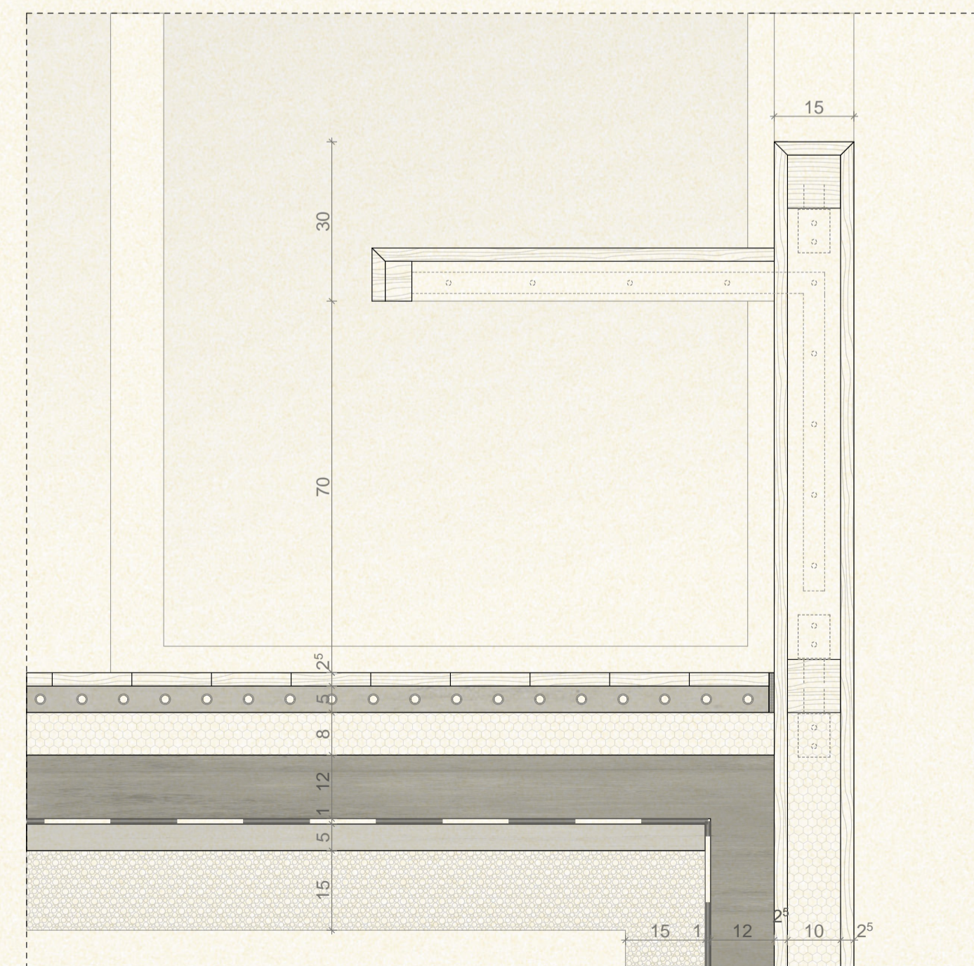
kóstoló mellvédkorlátjának kialakítása
