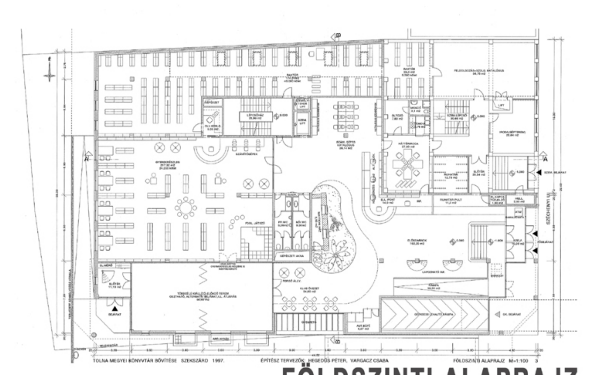
FÖLDSZINTI ALAPRAJZ
