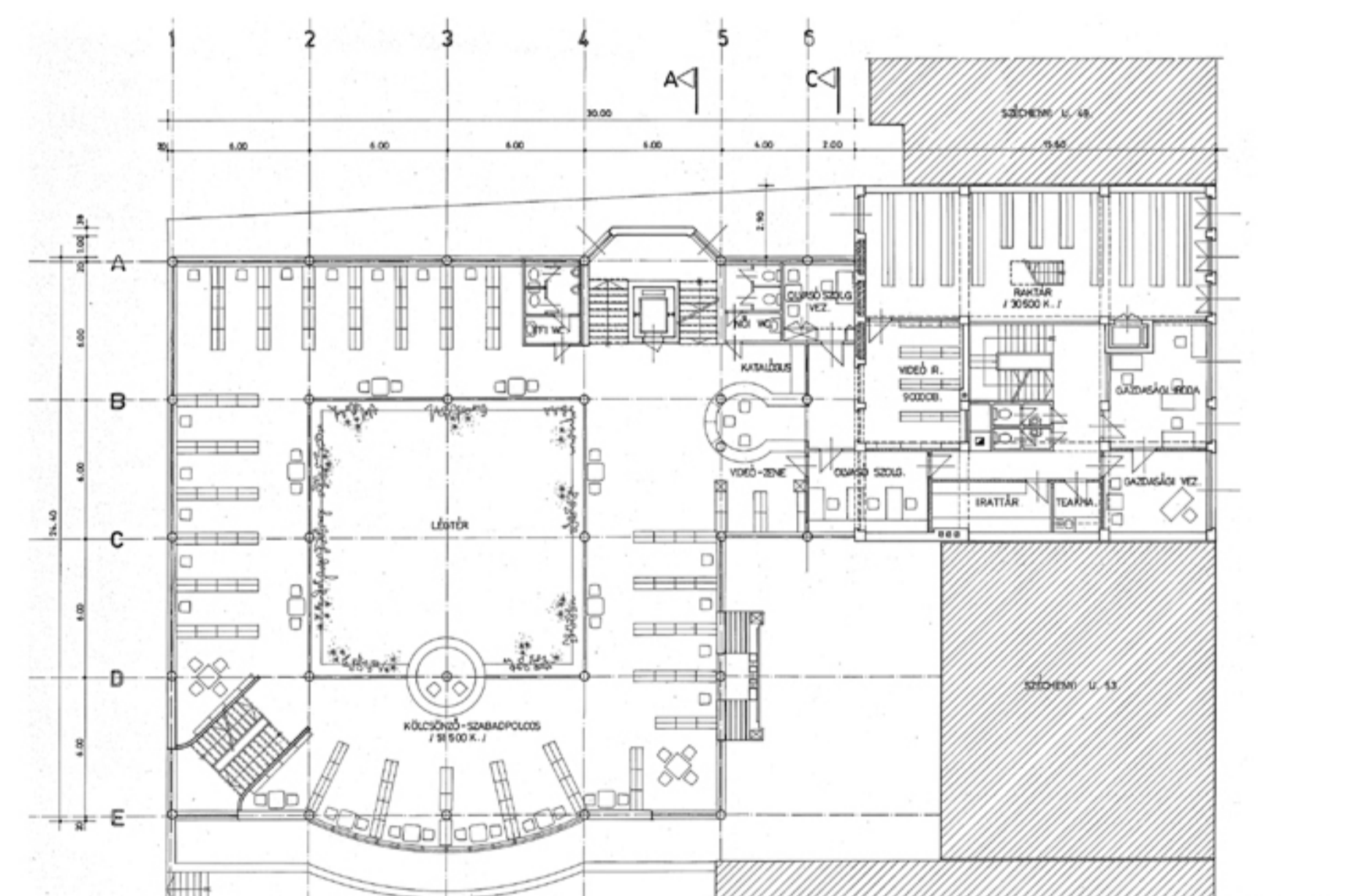
1. EMELETI ALAPRAJZ
