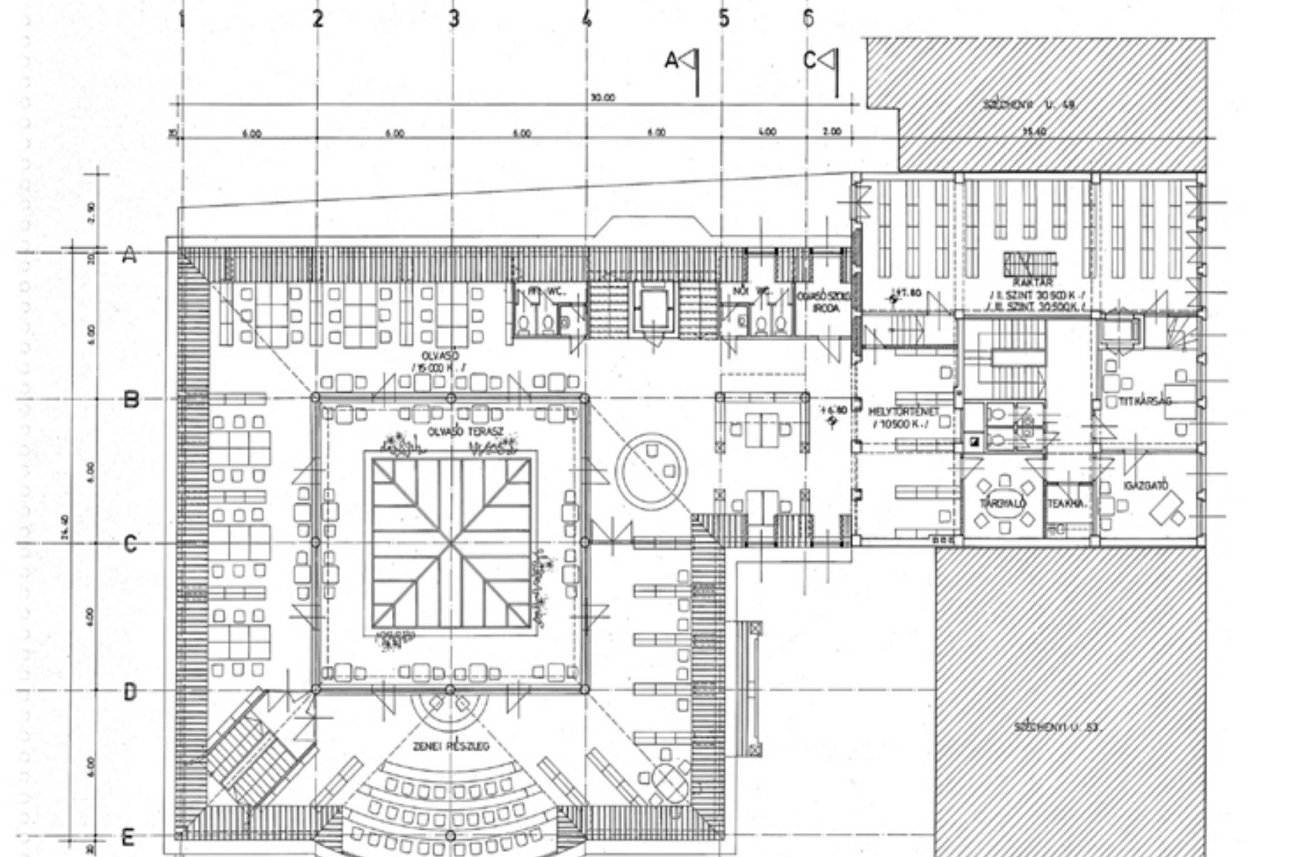
2. EMELETI ALAPRAJZ
