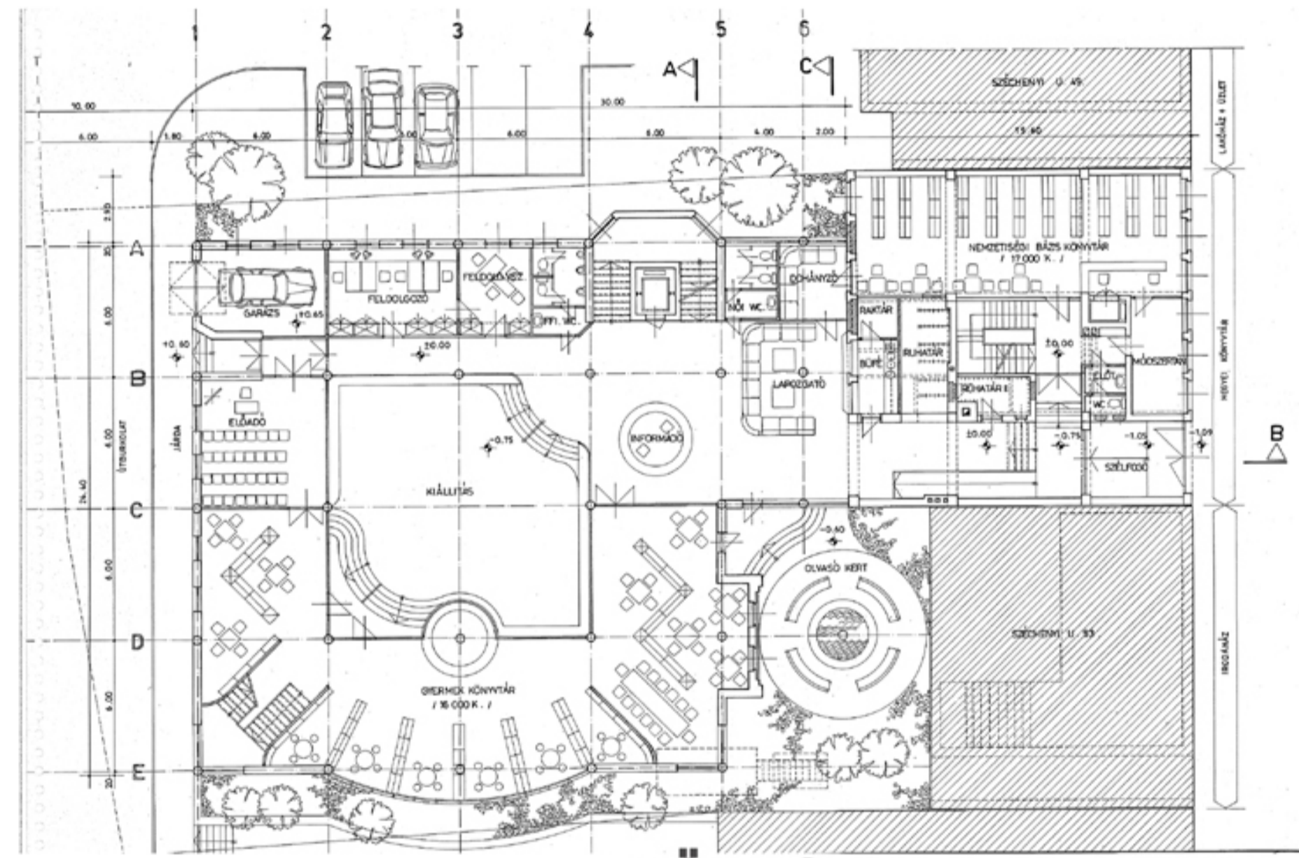
FÖLDSZINTI ALAPRAJZ
