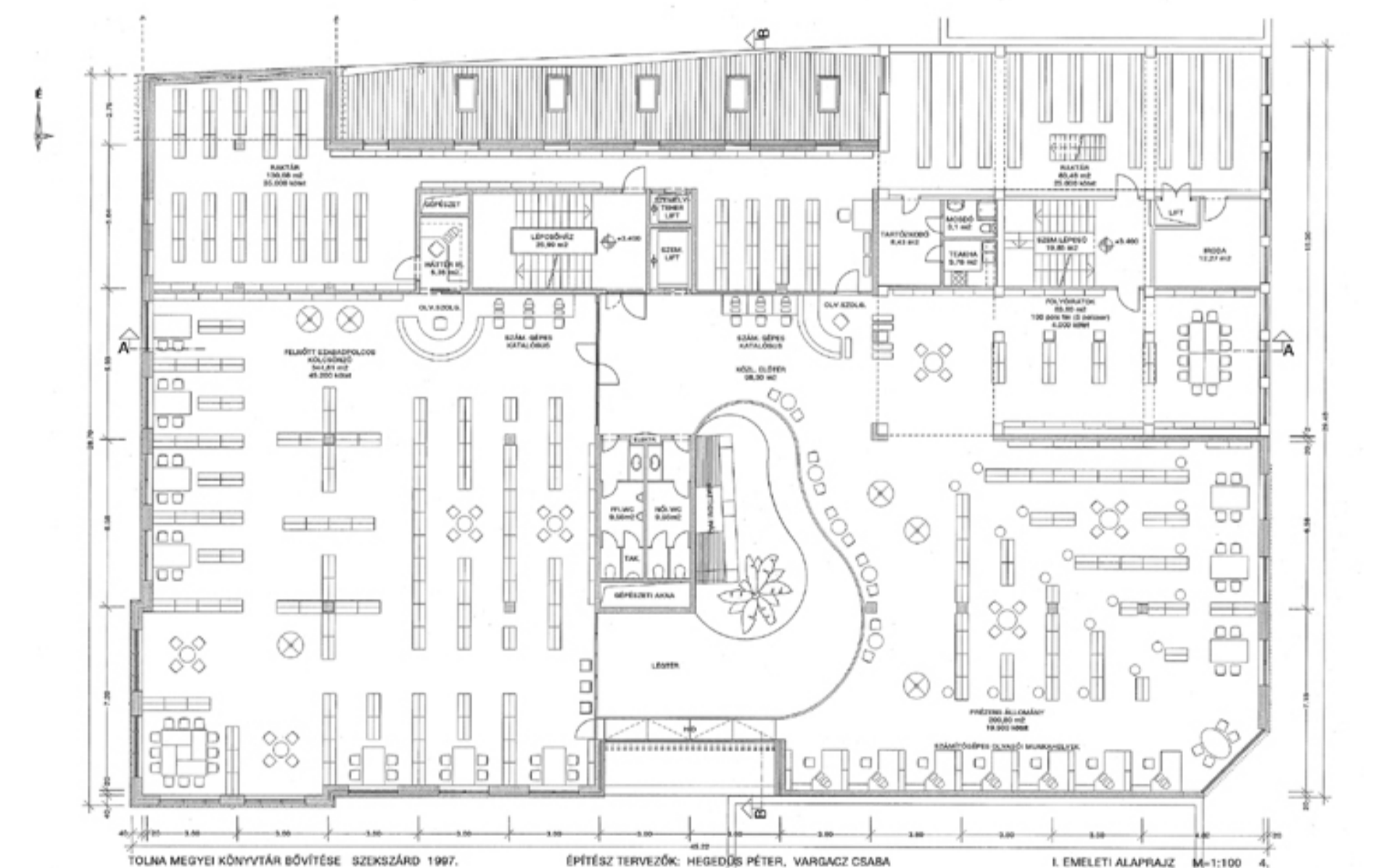
1. EMELETI ALAPRAJZ
