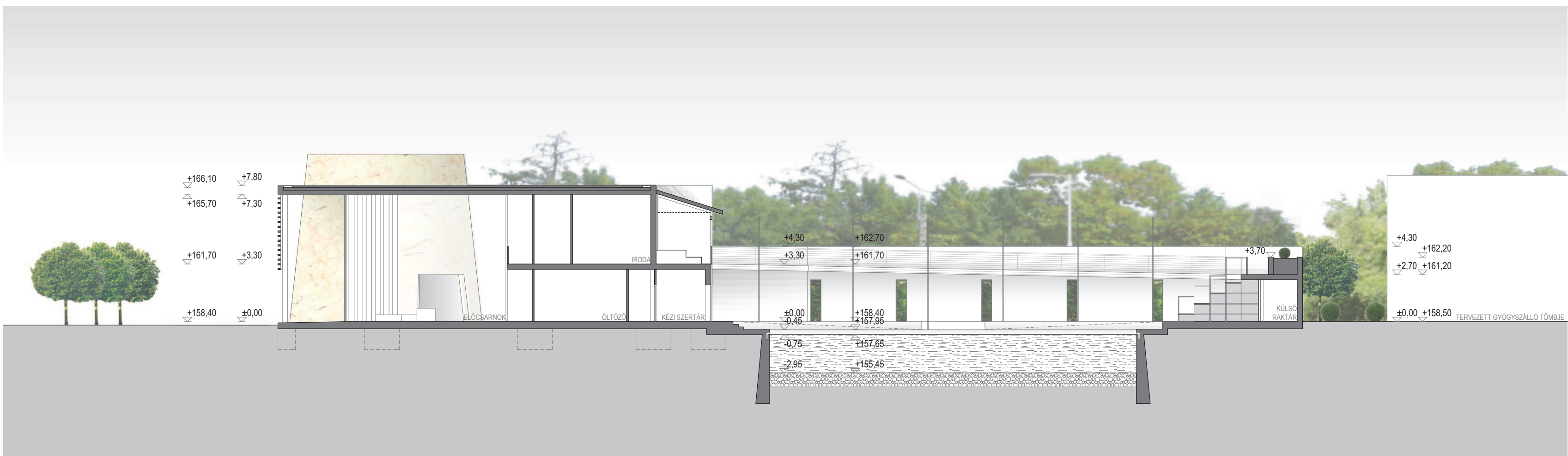
B-B METSZET
